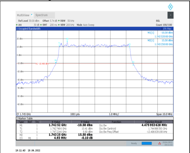
1-N66-PC3-15-5-M-1-DFT-QPSK-Outer_Full-25@0-Ant0-4.476-4.930-≤5-PASS
