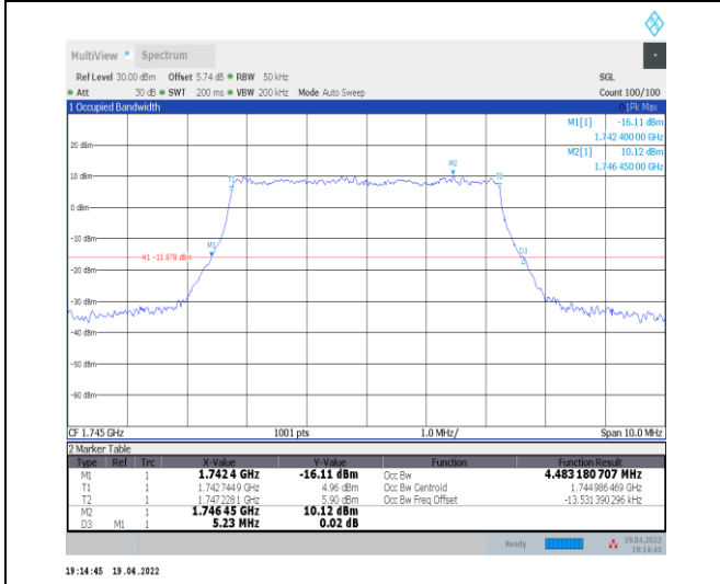
1-N66-PC3-15-5-M-6-CP-QPSK-Outer_Full-25@0-A nt0-4.483-5.230-≤5-PASS
