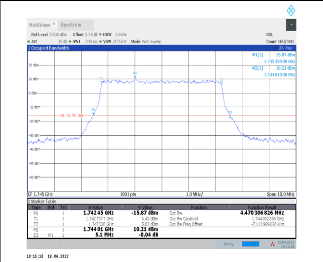
1-N66-PC3-15-5-M-7-CP-16QAM-Outer_Full-25@0- Ant0-4.47-5.100-≤5-PASS
