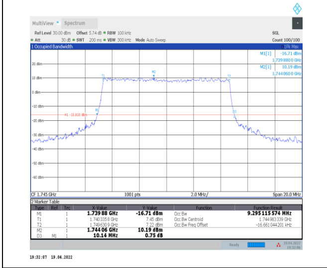
1-N66-PC3-15-10-M-7-CP-16QAM-Outer_Full-52 @ 0-Ant0-9.295-10.140-≤10-PASS
