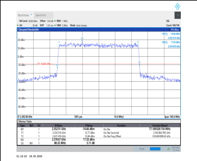
1-N41-PC1-30-80-M-1-DFT-QPSK-Outer_Full-216@ 0-Ant0-77.1-80.320-≤80-PASS
