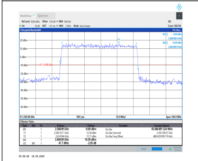
1-N41-PC1-30-50-M-1-DFT-QPSK-Outer_Full-128@ 0-Ant0-45.687-47.700-≤50-PASS
