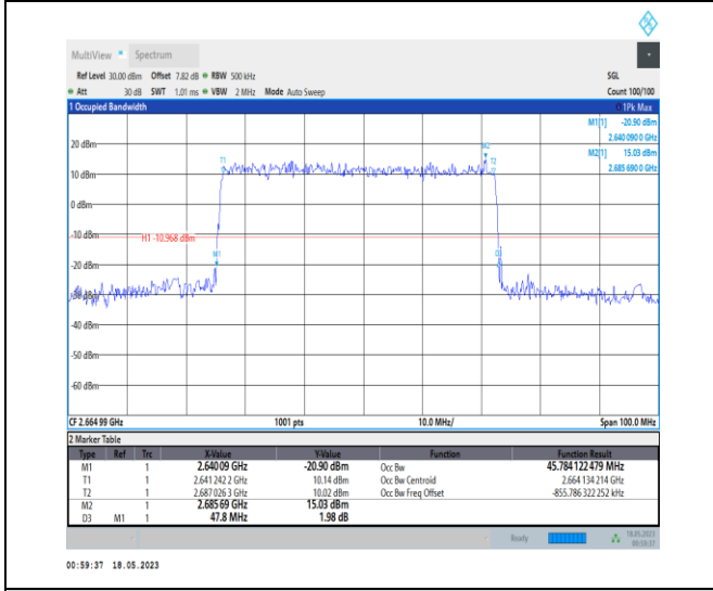
1-N41-PC1-30-50-H-4-DFT-64QAM-Outer_Full-128 @0-Ant0-45.784-47.800-≤50-PASS
