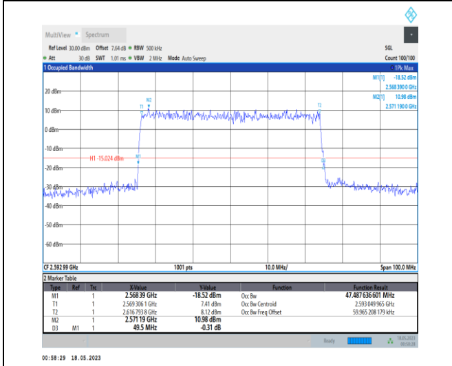
1-N41-PC1-30-50-M-9-CP-256QAM-Outer_Full-133 @0-Ant0-47.488-49.500-≤50-PASS
