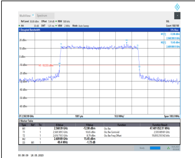
1-N41-PC1-30-50-M-7-CP-16QAM-Outer_Full-133@ 0-Ant0-47.401-49.400-≤50-PASS
