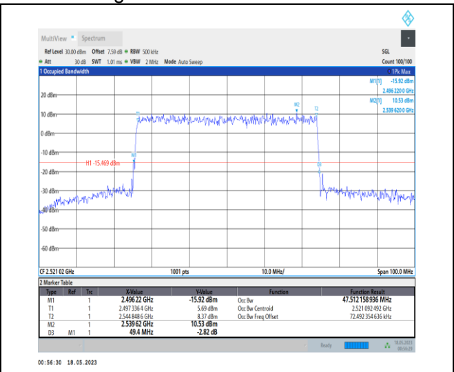
1-N41-PC1-30-50-L-9-CP-256QAM-Outer_Full-133 @0-Ant0-47.512-49.400-≤50-PASS
