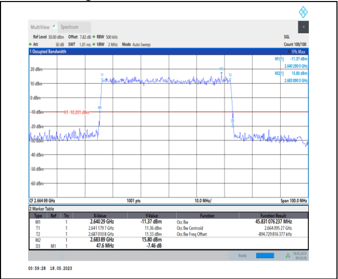
1-N41-PC1-30-50-H-3-DFT-16QAM-Outer_Full-128 @0-Ant0-45.831-47.600-≤50-PASS
