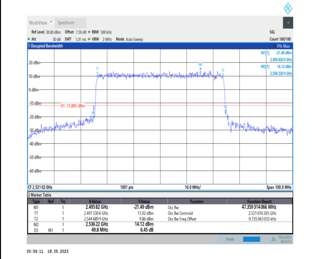
1-N41-PC1-30-50-L-7-CP-16QAM-Outer_Full-133@ 0-Ant0-47.359-49.800-≤50-PASS
