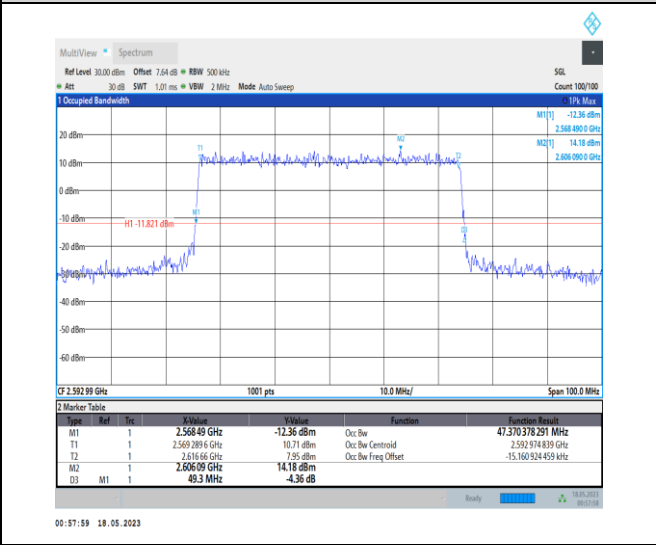
1-N41-PC1-30-50-M-6-CP-QPSK-Outer_Full-133 @ 0-Ant0-47.37-49.300-≤50-PASS
