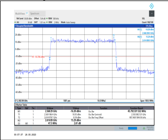
1-N41-PC1-30-50-M-4-DFT-64QAM-Outer_Full-128 @ 0-Ant0-45.792-47.500-≤50-PASS
