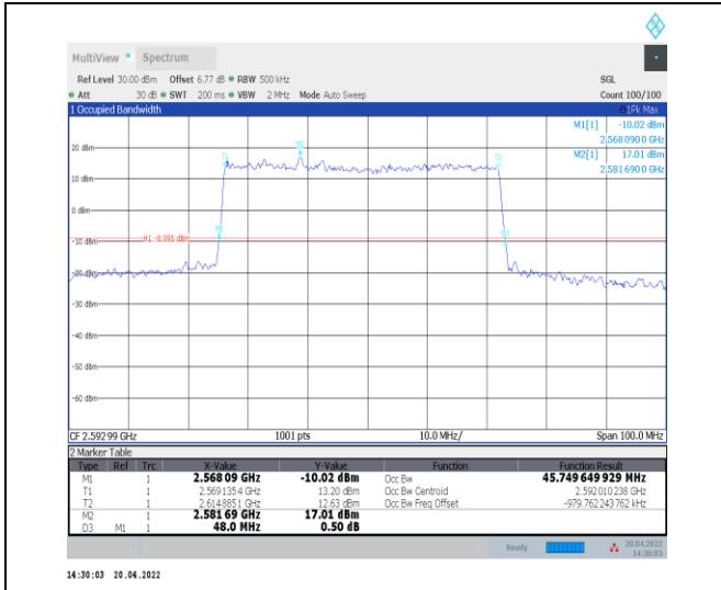
1-N41--30-50-M-3-DFT-16QAM-Outer_Full-128@0-A Ant0-45.75-48.000-≤50-PASS
