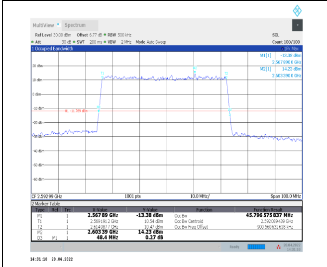
1-N41--30-50-M-5-DFT-256QAM-Outer_Full-128@0-A Ant0-45.797-48.400-≤50-PASS
