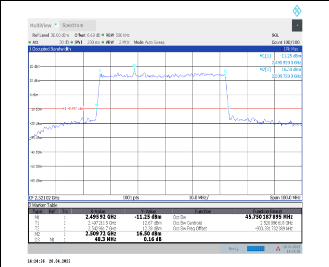
1-N41--30-50-L-3-DFT-16QAM-Outer_Full-128@0-A nt0-45.75-48.300-≤50-PASS
