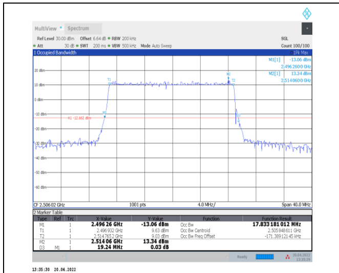
1-N41--30-20-L-5-DFT-256QAM-Outer_Full-50@0-A nt0-17.833-19.240-≤20-PASS
