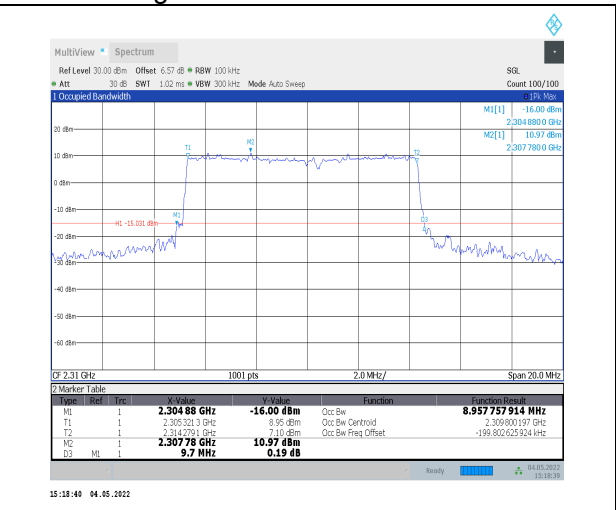
1-N30--15-10-L-3-DFT-16QAM-Outer_Full-50@0-Ant 0-8.958-9.700-≤10-PASS
