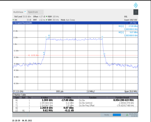
1-N30--15-10-L-5-DFT-256QAM-Outer_Full-50@0-A nt0-8.954-9.620-≤10-PASS
