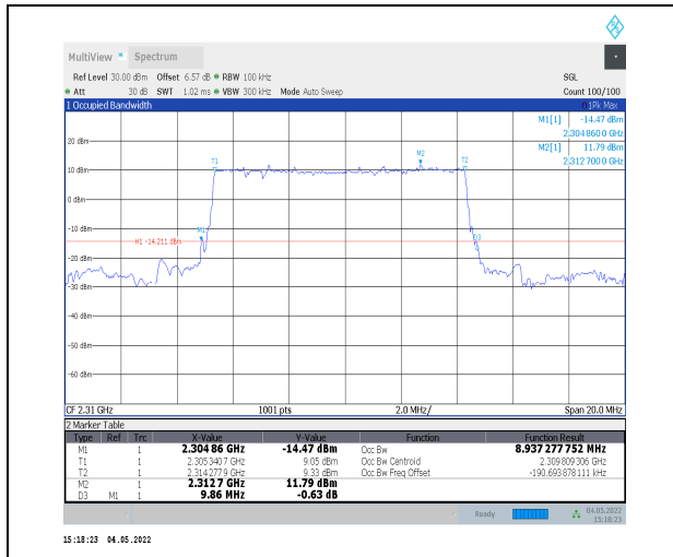
1-N30--15-10-L-2-DFT-PI2BPSK-Outer_Full-50@0-A nt0-8.937-9.860-≤10-PASS
