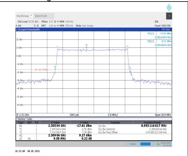
1-N30--15-10-H-5-DFT-256QAM-Outer_Full-50@0-A nt0-8.955-9.580-≤10-PASS
