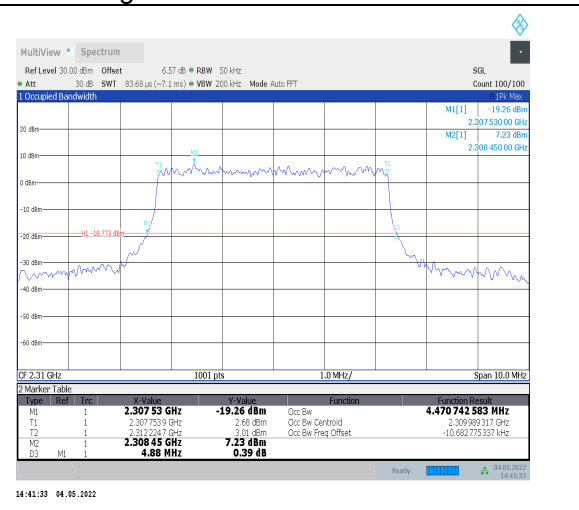
1-N30--15-5-M-9-CP-256QAM-Outer_Full-25@0-Ant 0-4.471-4.880≤5-PASS
