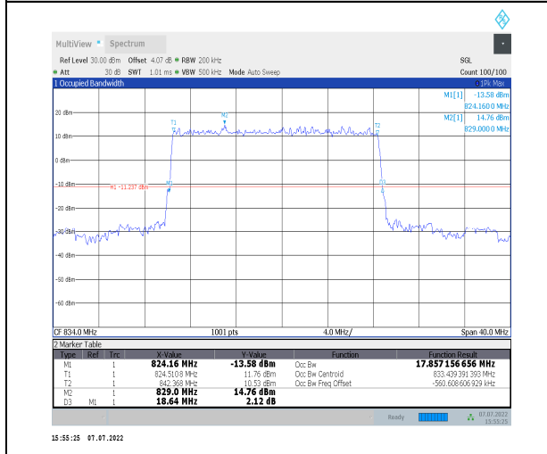
1-N26-824-849--15-20-L-2-DFT-P12BPSK-Outer_Full-100@0-Ant0-17.857-18.640-≤20-PASS
