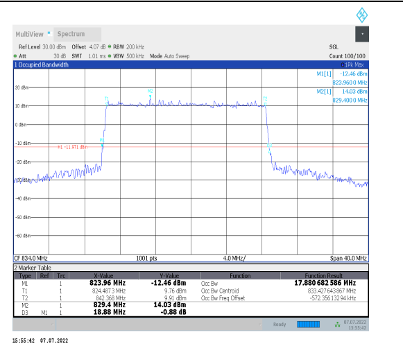
1-N26-824-849--15-20-L-3-DFT-16QAM-Outer_Full-100@0-Ant0-17.881-18.880-≤20-PASS
