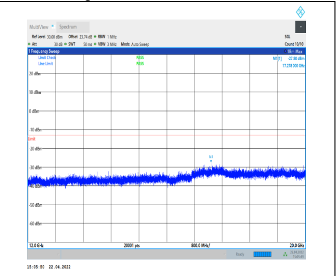
1-N25--15-40-L-1-DFT-PI2BPSK-Inner_1RB_Left-1 @ 1-12000-20000-Ant0--27.80--13-PASS
