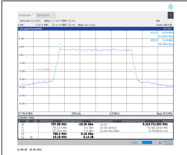
1-N14--15-10-M-9-CP-256QAM-Outer_Full-52@0-A nt0-9.317-10.180-<math>\leq 10</math>-PASS
