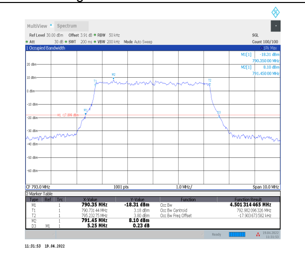
1-N14--15-5-M-9-CP-256QAM-Outer_Full-25@0-Ant 0-4.501-5.250-≤5-PASS
