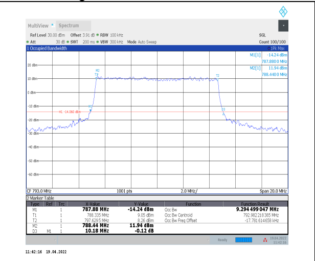
1-N14--15-10-L-7-CP-16QAM-Outer_Full-52@0-Ant0 -9.294-10.180≤10-PASS
