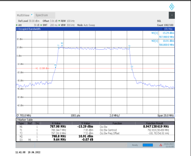
1-N14--15-10-L-5-DFT-256QAM-Outer_Full-50@0-A nt0-8.947-9.640≤10-PASS
