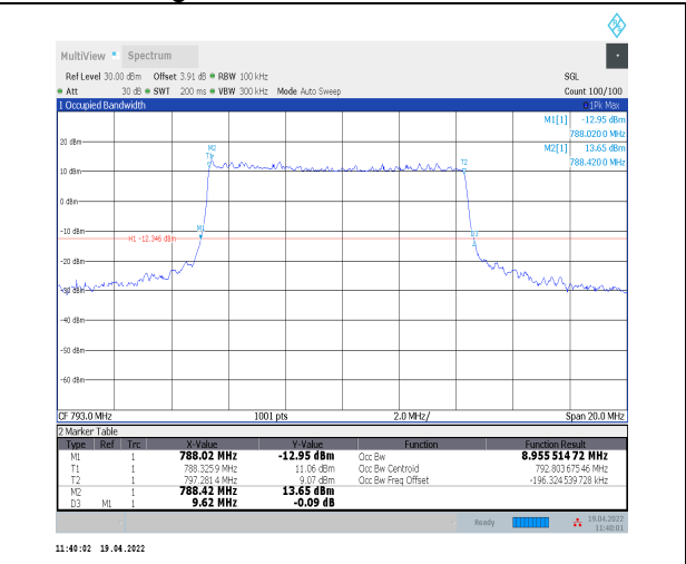
1-N14--15-10-L-3-DFT-16QAM-Outer_Full-50@0-Ant 0-8.956-9.620≤10-PASS
