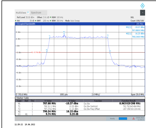
1-N14--15-10-L-2-DFT-PI2BPSK-Outer_Full-50@0-A nt0-8.963-9.740≤10-PASS
