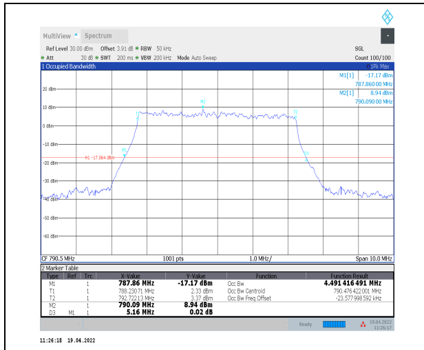
1-N14--15-5-L-9-CP-256QAM-Outer_Full-25@0-Ant 0-4.491-5.160-≤5-PASS
