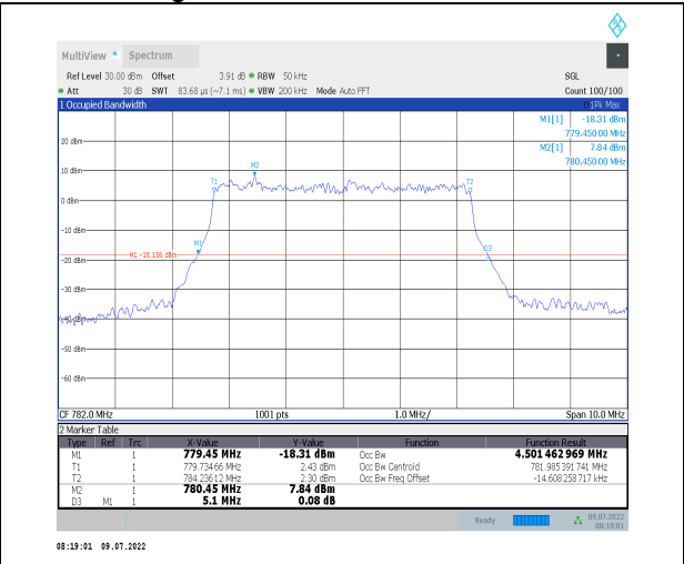
1-N13--15-5-M-9-CP-256QAM-Outer_Full-25@0-Ant 0-4.501-5.100-≤5-PASS
