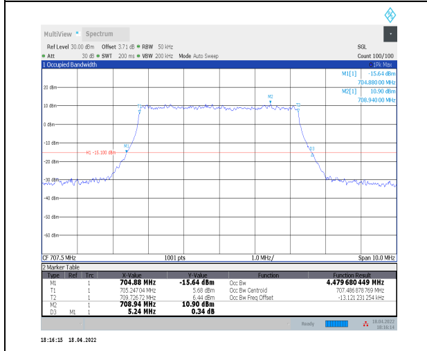
1-N12--15-5-M-6-CP-QPSK-Outer_Full-25@0-Ant0-4 .48-5.240-≤5-PASS
