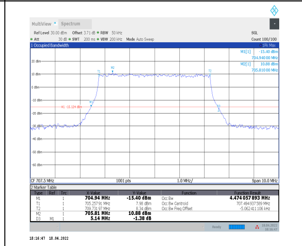
1-N12--15-5-M-7-CP-16QAM-Outer_Full-25@0-Ant0 -4.474-5.140-≤5-PASS
