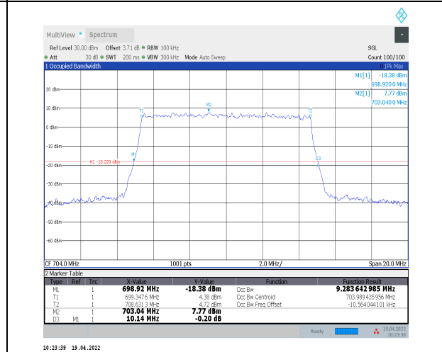
1-N12--15-10-L-9-CP-256QAM-Outer_Full-52@0-An 10-9.284-10.140≤10-PASS
