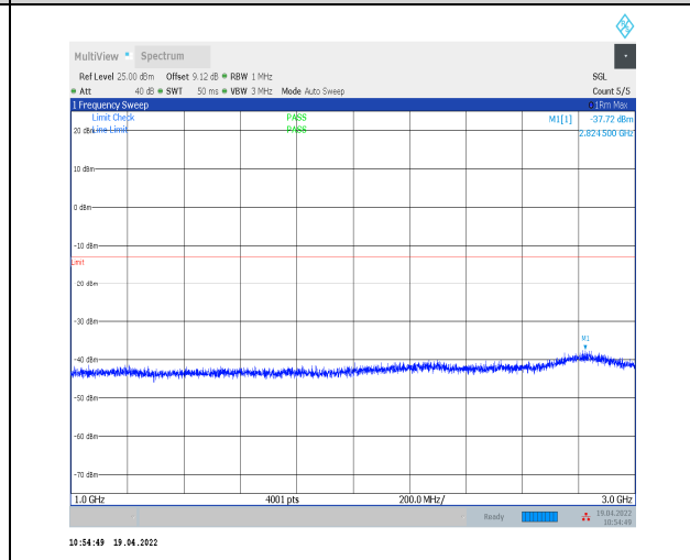
1-N12--15-15-H-1-DFT-PI2BPSK-Inner_1RB_Left-1 @1-1000-3000-Ant0--37.72--13-PASS
