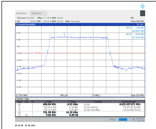
1-N12--15-10-L-2-DFT-PI2BPSK-Outer_Full-50@0-A nt0-8.931-9.660-≤10-PASS
