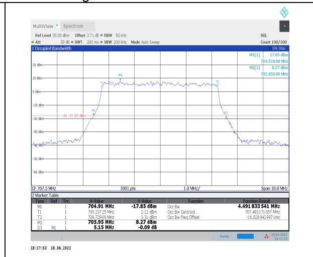
1-N12--15-5-M-9-CP-256QAM-Outer_Full-25@0-Ant 0-4.492-5.150-≤5-PASS
