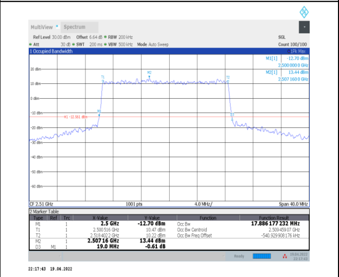
1-N7--15-20-L-3-DFT-16QAM-Outer_Full-100@0-Ant 0-17.886-19.000-≤20-PASS
