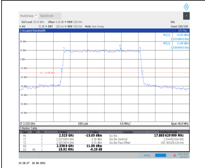
1-N7--15-20-M-5-DFT-256QAM-Outer_Full-100@0-A nt0-17.886-18.920-≤20-PASS
