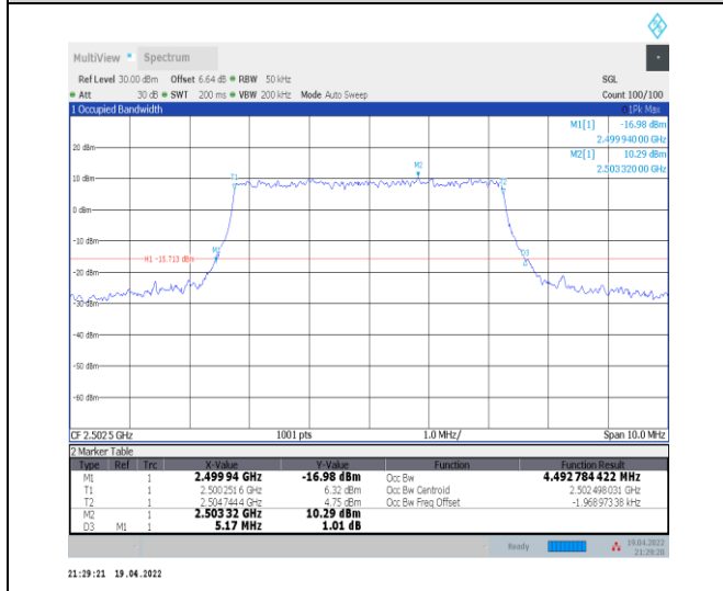
1-N7--15-5-L-7-CP-16QAM-Outer_Full-25@0-Ant0-4 .493-5.170-≤5-PASS
