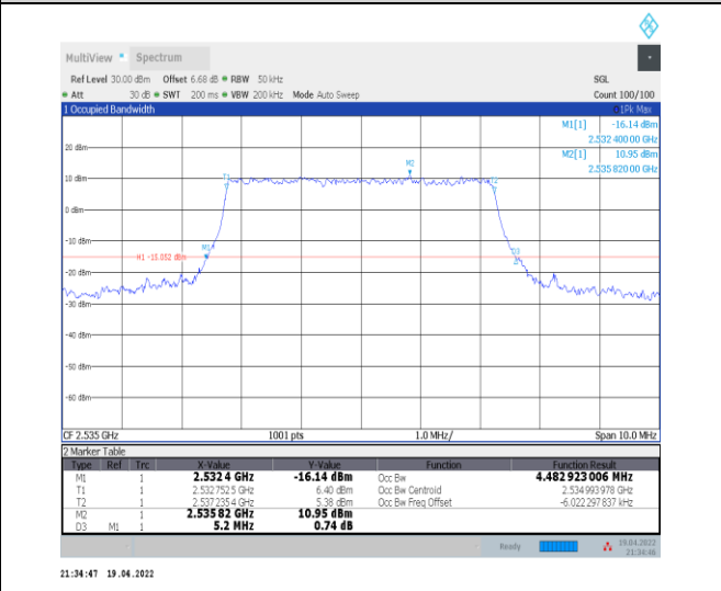
1-N7--15-5-M-7-CP-16QAM-Outer_Full-25@0-Ant0- 4.483-5.200-≤5-PASS
