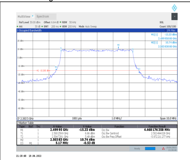
1-N7--15-5-L-6-CP-QPSK-Outer_Full-25@0-Ant0-4. 468-5.170-≤5-PASS
