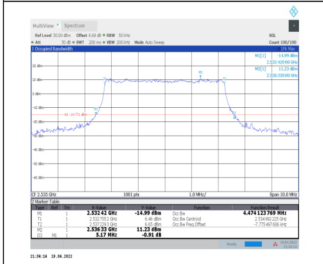
1-N7--15-5-M-6-CP-QPSK-Outer_Full-25@0-Ant0-4. 474-5.170-≤5-PASS
