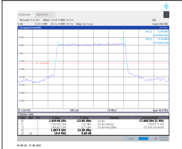
1-N2--15-20-L-2-DFT-PI2BPSK-Outer_Full-100@0-A nt0-17.86-19.000≤20-PASS
