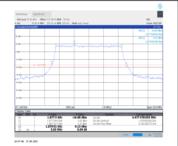
1-N2--15-5-M-7-CP-16QAM-Outer_Full-25@0-Ant0- 4.477-5.050≤5-PASS
