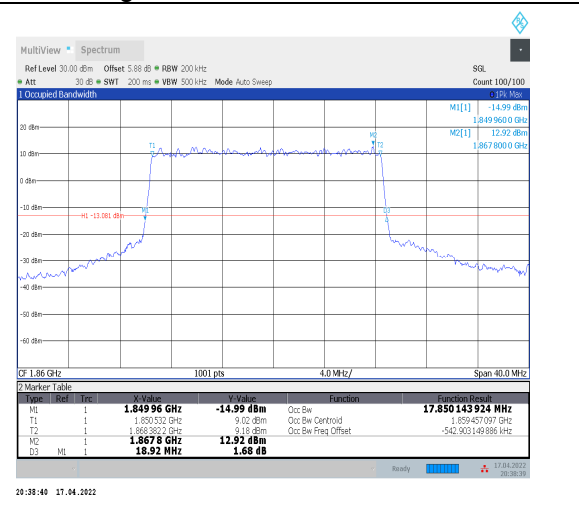
1-N2--15-20-L-1-DFT-QPSK-Outer_Full-100@0-Ant0 -17.85-18.920≤20-PASS
