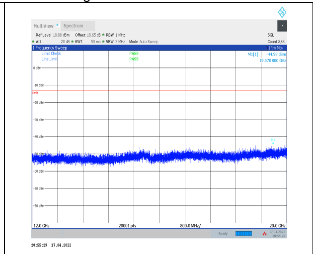
1-N2--15-20-L-1-DFT-PI2BPSK-Inner_1RB_Left-1@1 -12000-20000-Ant0--44.98--13-PASS
