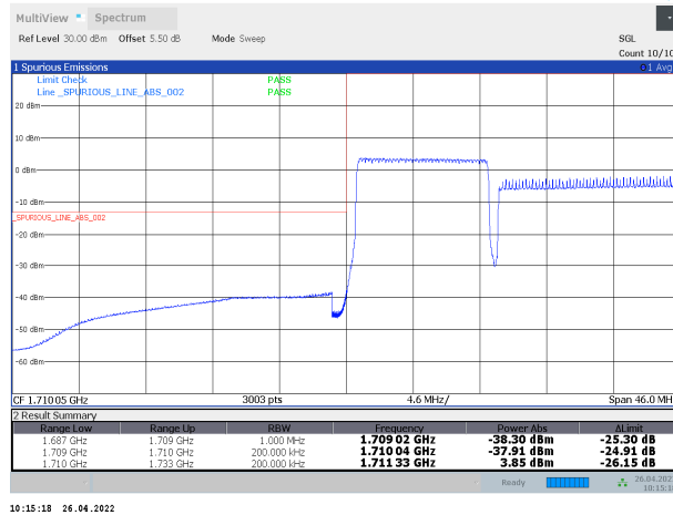
66-66-10MHz-15MHz-QPSK-QPSK-132025-132145-50RB#0-75RB#0
