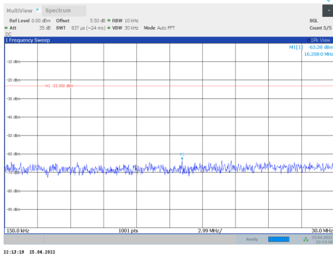
2-2-20MHz-20MHz-QPSK-QPSK-18700-18898-1RB#0-0RB#0-0.15~30MHz
