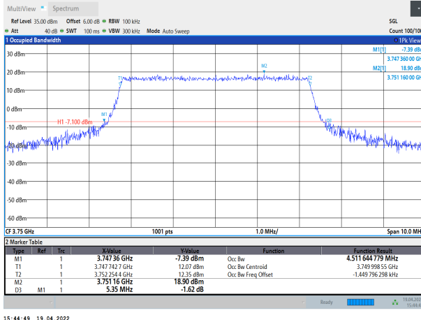
Band43-5MHz-QPSK-45090-25RB#0
