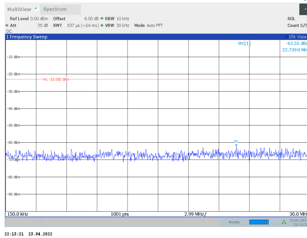
Band43-20MHz-QPSK-44690-1RB#0-Range2:0.15~30MHz
