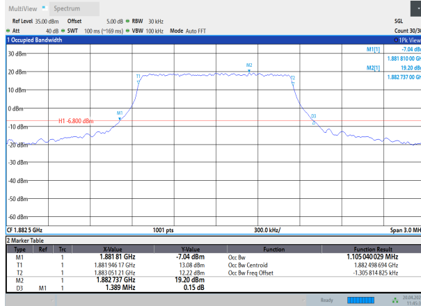
Band25-1.4MHz-QPSK-26365-6RB#0
