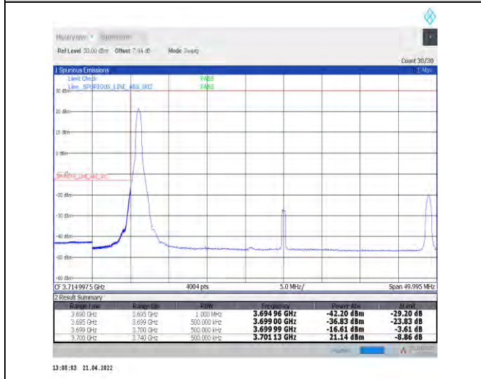
1-N78-3700-3800--30-40-L-4-CP-QPSK-Edge_1RB_L eft-1@0-Ant0-PASS-see graph
