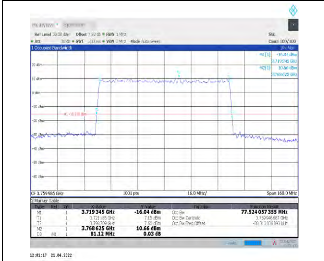
1-N78-3700-3800--30-80-H-9-CP-256QAM-Outer_Fu ll-217@0-Ant0-77.524-81.120-≤80-PASS
