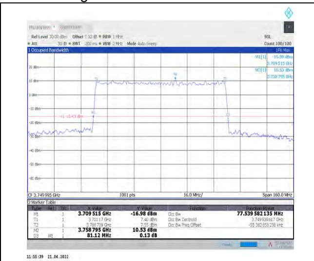
1-N78-3700-3800--30-80-M-9-CP-256QAM-Outer_Full -217@0-Ant0-77.54-81.120-≤80-PASS
