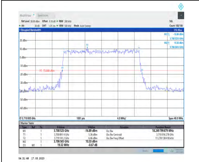
1-N78-3700-3800-PC1-30-20-L-9-CP-256QAM-Outer _Full-51@0-Ant0-18.25-19.320-≤20-PASS
