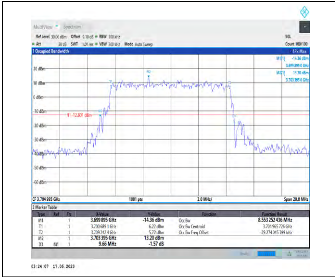
1-N78-3700-3800-PC1-30-10-L-5-DFT-256QAM-Out er_Full-24@0-Ant0-8.553-9.660-≤10-PASS
