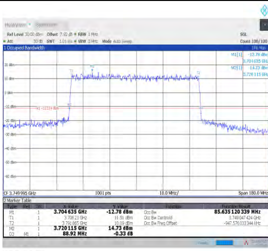
1-N78-3700-3800--30-90-M-1-DFT-QPSK-Outer_Full -240@0-Ant0-85.635-88.920-≤90-PASS
