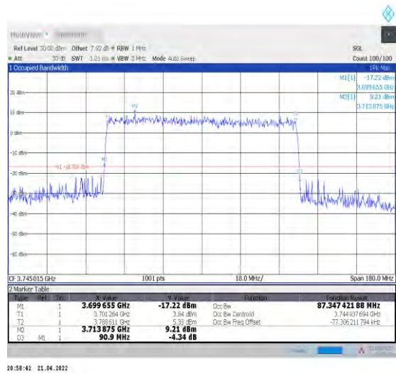
1-N78-3700-3800--30-90-L-9-CP-256QAM-Outer_Fu ll-245@0-Ant0-87.347-90.900-<=90-PASS
