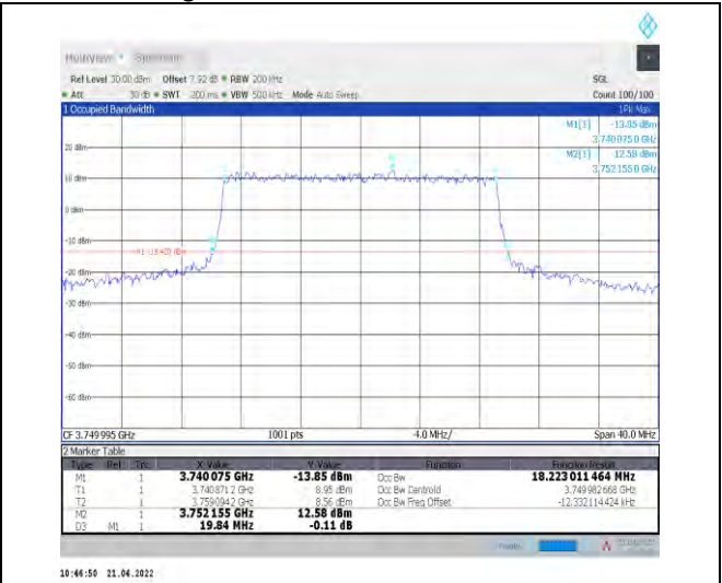
1-N78-3700-3800--30-20-M-7-CP-16QAM-Outer_Full-51@0-Ant0-18.223-19.840-≤20-PASS
