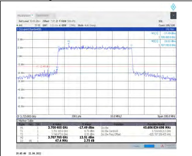
1-N78-3700-3800--30-50-L-3-DFT-16QAM-Outer_Fu ll-128@0-Ant0-45.607-47.400-<math>\leq 50</math>-PASS
