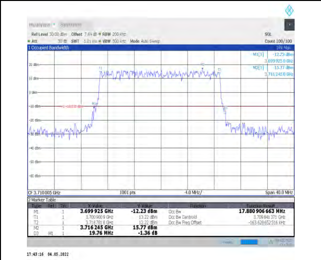
1-N78-3700-3800--30-20-L-2-DFT-PI2BPSK-Outer_Full-50@0-Ant0-17.881-19.760-≤20-PASS
