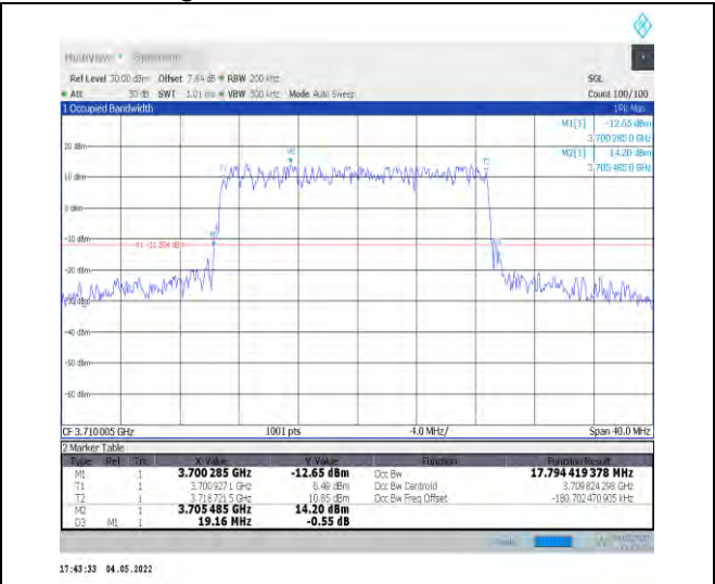
1-N78-3700-3800--30-20-L-4-DFT-64QAM-Outer_Fu II-50@0-Ant0-17.794-19.160-<=20-PASS
