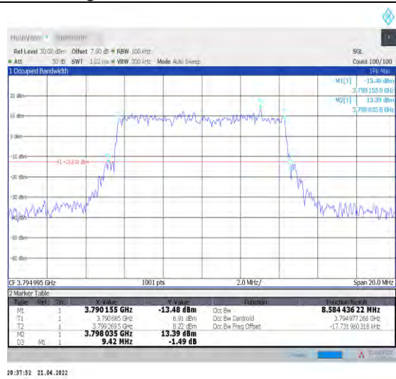
1-N78-3700-3800--30-10-H-4-DFT-64QAM-Outer_Fu II-24@0-Ant0-8.584-9.420-≤10-PASS
