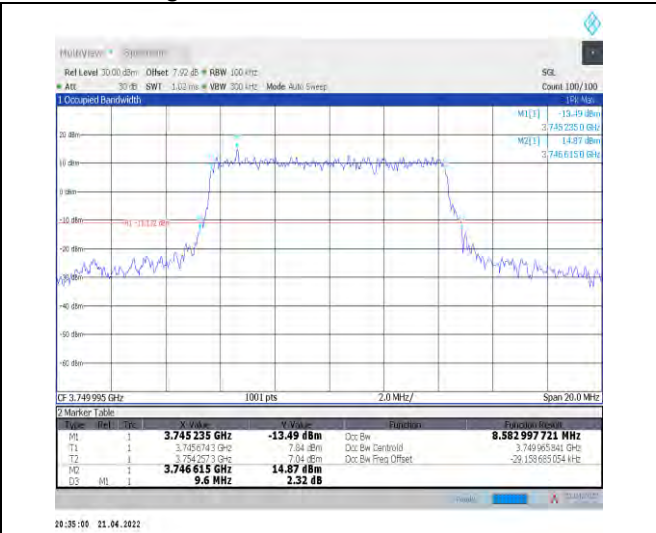
1-N78-3700-3800--30-10-M-1-DFT-QPSK-Outer_Full -24@0-Ant0-8.583-9.600-≤10-PASS
