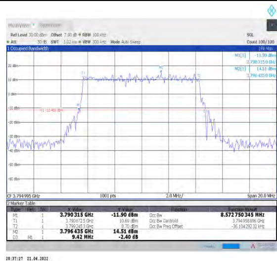
1-N78-3700-3800--30-10-H-2-DFT-PI2BPSK-Outer_Full -24@0-Ant0-8.573-9.420-≤10-PASS
