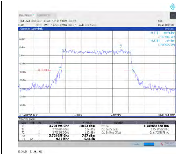
1-N78-3700-3800--30-10-L-9-CP-256QAM-Outer_Fu II-24@0-Ant0-8.55-9.320-≤10-PASS
