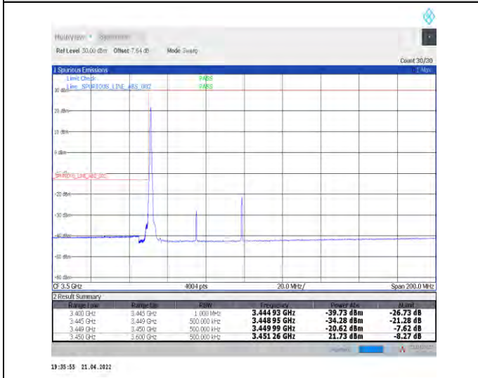
1-N78-3450-3550--30-50-L-4-CP-QPSK-Edge_1RB_L eft-1@0-Ant0-PASS-see graph
