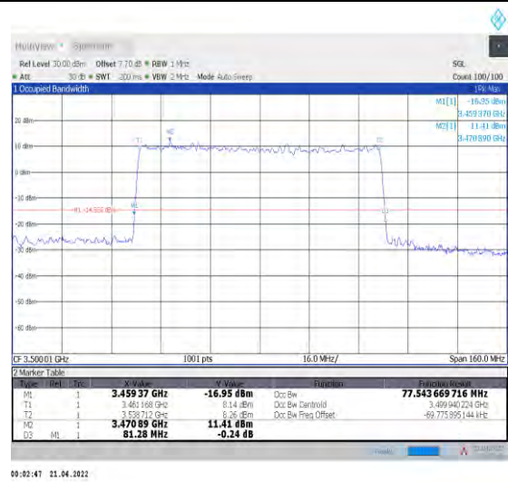
1-N78-3450-3550--30-80-M-9-CP-256QAM-Outer_Full -217@0-Ant0-77.544-81.280-≤80-PASS
