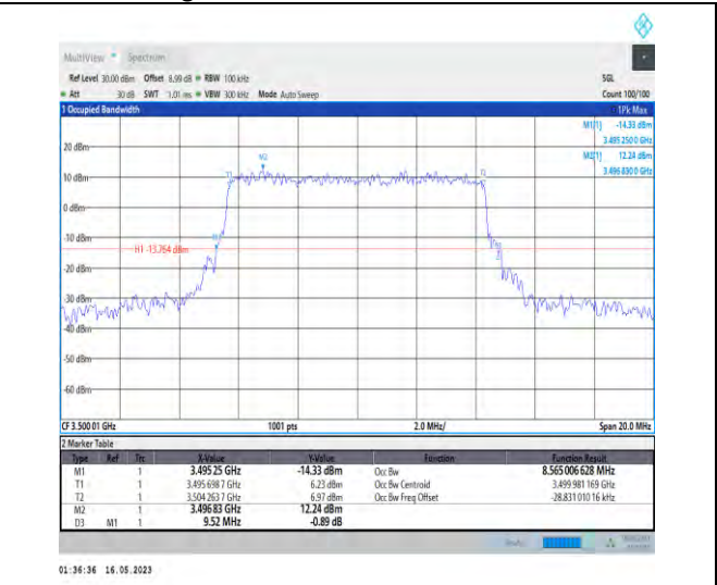
1-N78-3450-3550-PC1-30-10-M-5-DFT-256QAM-Out er_Full-24@0-Ant0-8.565-9.520-≤10-PASS
