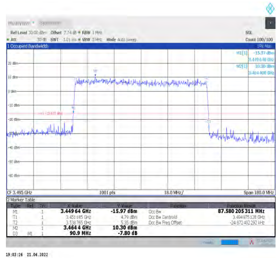
1-N78-3450-3550--30-90-L-9-CP-256QAM-Outer_Fu ll-245@0-Ant0-87.58-90.900≤90-PASS
