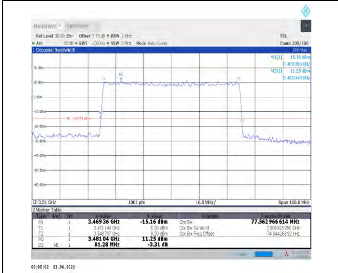
1-N78-3450-3550--30-80-H-9-CP-256QAM-Outer_Fu ll-217@0-Ant0-77.563-81.280-≤80-PASS
