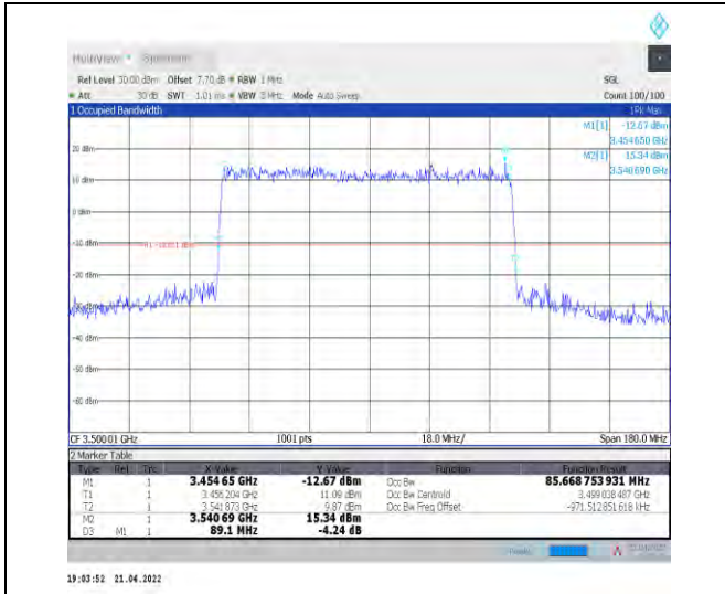
1-N78-3450-3550--30-90-M-1-DFT-QPSK-Outer_Full -240@0-Ant0-85.669-89.100-≤90-PASS
