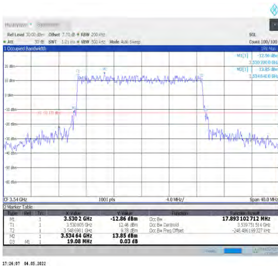
1-N78-3450-3550--30-20-H-3-DFT-16QAM-Outer_Fu II-50@0-Ant0-17.893-19.080-≤20-PASS
