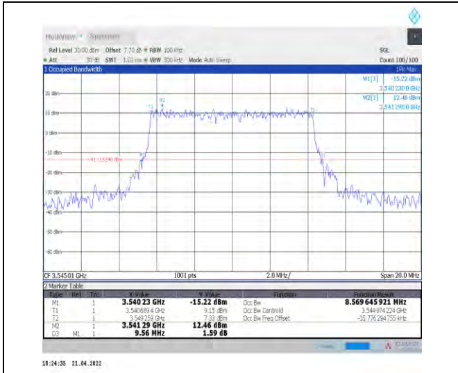
1-N78-3450-3550--30-10-H-3-DFT-16QAM-Outer_Fu Il-24@0-Ant0-8.57-9.560-≤10-PASS
