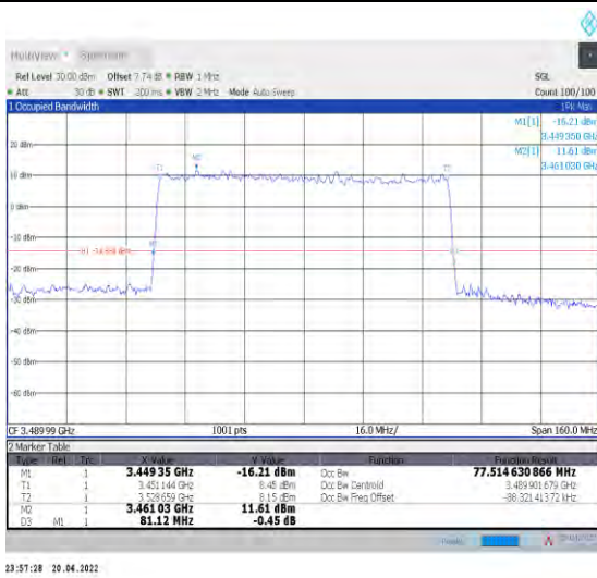
1-N78-3450-3550--30-80-L-9-CP-256QAM-Outer_Fu ll-217@0-Ant0-77.515-81.120≤80-PASS
