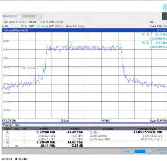
1-N78-3450-3550--30-20-H-1-DFT-QPSK-Outer_Full -50@0-Ant0-17.854-19.440-≤20-PASS
