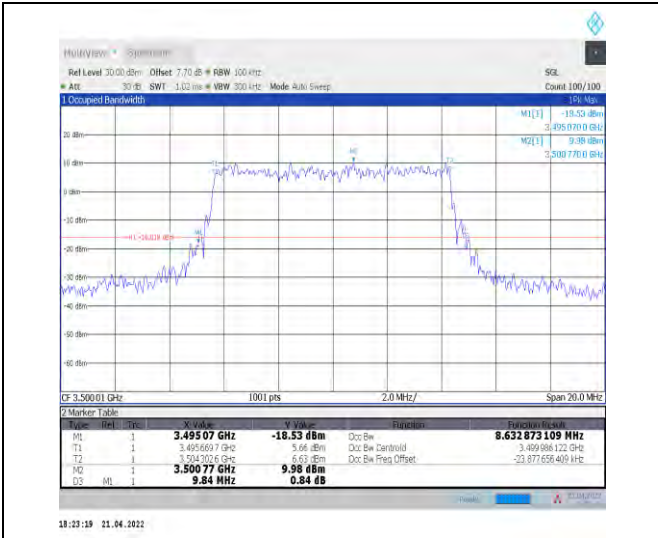
1-N78-3450-3550--30-10-M-8-CP-64QAM-Outer_Full -24@0-Ant0-8.633-9.840-≤10-PASS
