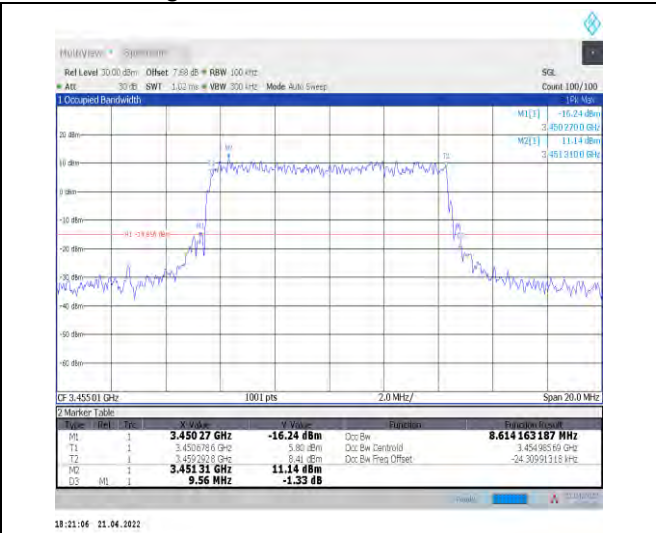
1-N78-3450-3550--30-10-L-6-CP-QPSK-Outer_Full-24@0-Ant0-8.614-9.560-≤10-PASS
