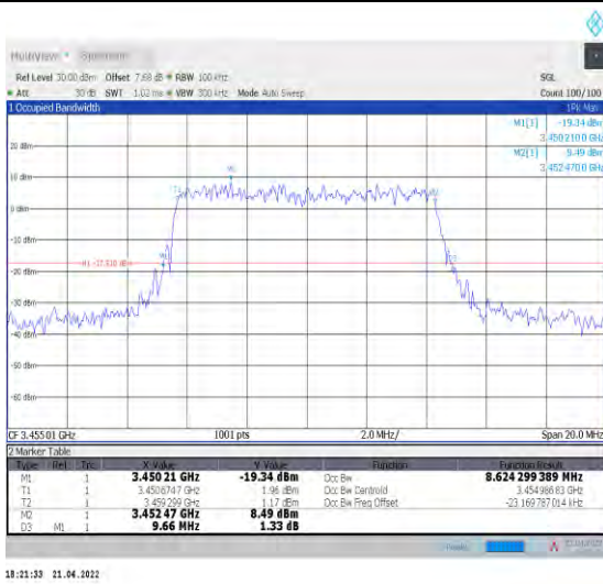
1-N78-3450-3550--30-10-L-9-CP-256QAM-Outer_Full-24@0-Ant0-8.624-9.660-≤10-PASS
