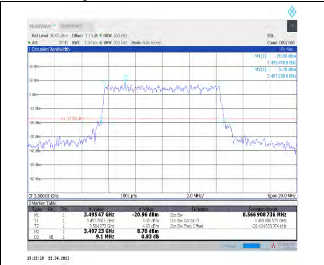
1-N78-3450-3550--30-10-M-9-CP-256QAM-Outer_Full -24@0-Ant0-8.567-9.100-≤10-PASS
