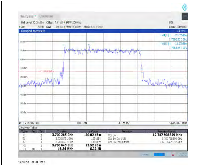
1-N77-3700-3980--30-20-L-3-DFT-16QAM-Outer_Fu ll-50@0-Ant0-17.788-18.840-<math>\leq 20</math>-PASS
