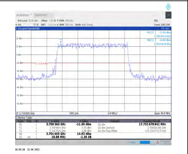
1-N77-3700-3980--30-20-L-2-DFT-PI2BPSK-Outer_Full ull-50@0-Ant0-17.753-18.880-≤20-PASS
