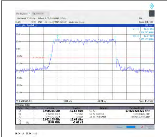
1-N77-3700-3980--30-20-H-1-DFT-QPSK-Outer_Full -50@0-Ant0-17.876-18.840-≤20-PASS
