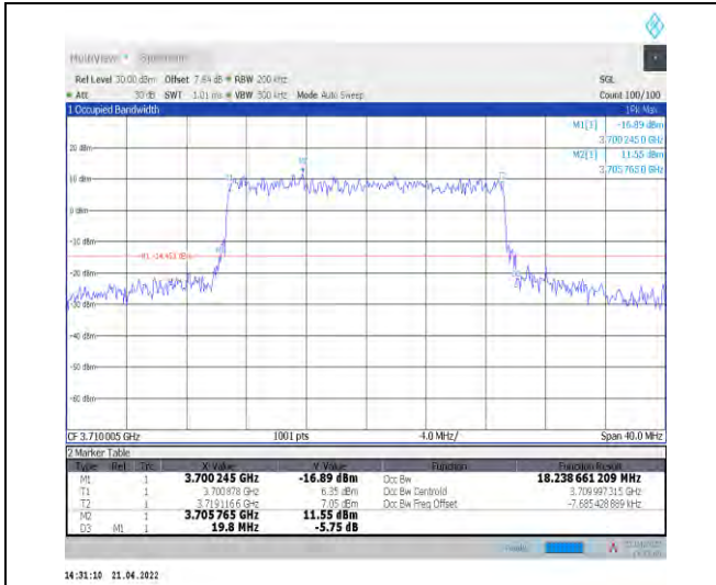
1-N77-3700-3980--30-20-L-7-CP-16QAM-Outer_Full -51@0-Ant0-18.239-19.800-≤20-PASS
