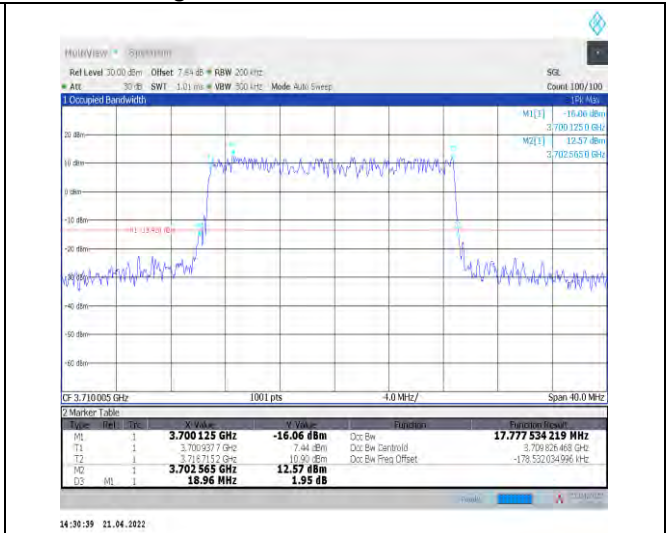
1-N77-3700-3980--30-20-L-4-DFT-64QAM-Outer_Fu ll-50@0-Ant0-17.778-18.960-<math>\leq 20</math>-PASS
