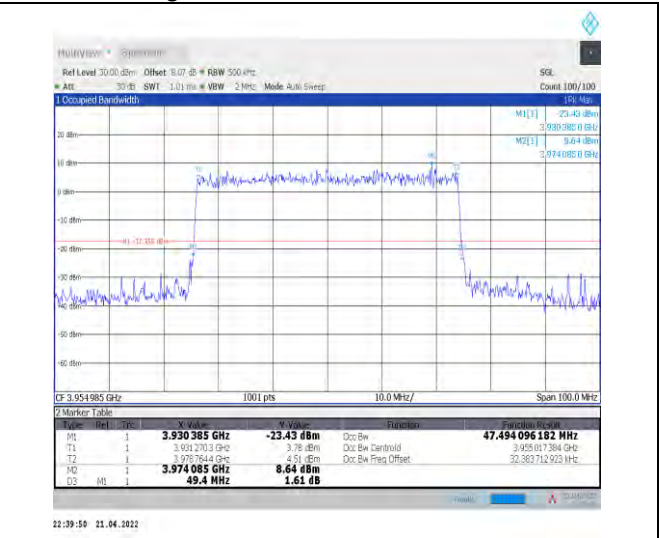
1-N77-3700-3980--30-50-H-9-CP-256QAM-Outer_Fu ll-133@0-Ant0-47.494-49.400-≤50-PASS
