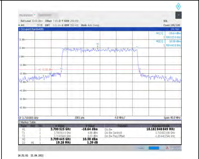
1-N77-3700-3980--30-20-L-6-CP-QPSK-Outer_Fu ll-50@0-Ant0-18.183-19.280-<math>\leq 20</math>-PASS
