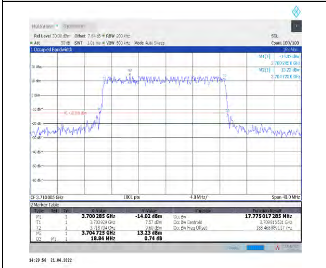
1-N77-3700-3980--30-20-L-1-DFT-QPSK-Outer_Full -50@0-Ant0-17.775-18.840-≤20-PASS
