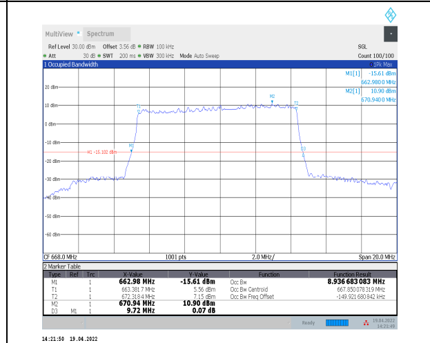
1-N71--15-10-L-5-DFT-256QAM-Outer_Full-50@0-A nt0-8.937-9.720-≤10-PASS
