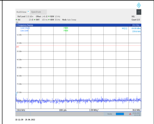
1-N71--15-20-M-1-DFT-PI2BPSK-Inner_1RB_Left-1 @1-0.15-30-Ant0--84.08--23-PASS
