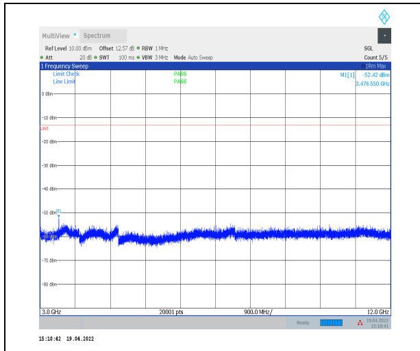
1-N71--15-20-L-1-DFT-PI2BPSK-Inner_1RB_Left-1 @1-3000-12000-Ant0--52.42--13-PASS
