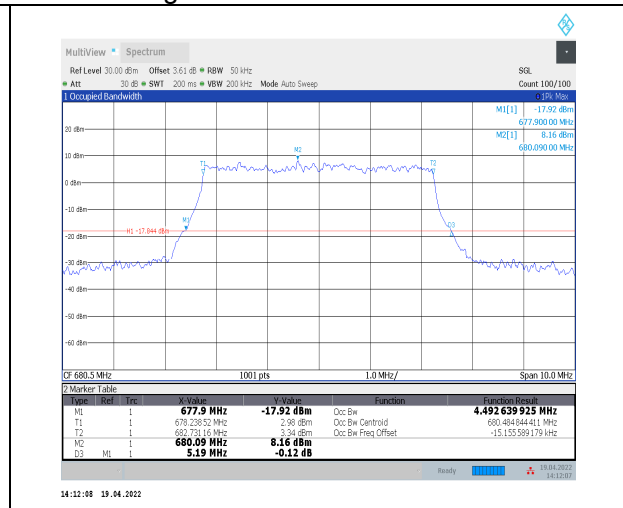
1-N71--15-5-M-9-CP-256QAM-Outer_Full-25@0-Ant 0-4.493-5.190≤5-PASS
