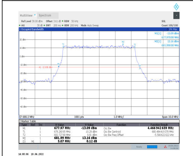
1-N71--15-5-M-2-DFT-PI2BPSK-Outer_Full-25@0-A nt0-4.467-5.070-≤5-PASS
