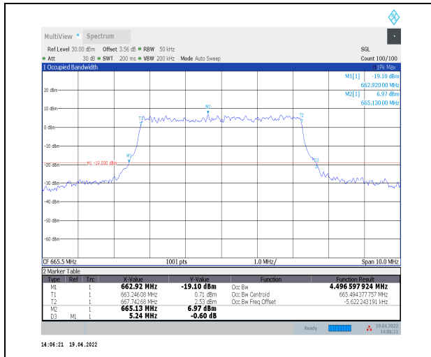
1-N71--15-5-L-9-CP-256QAM-Outer_Full-25@0-Ant0 -4.497-5.240-≤5-PASS
