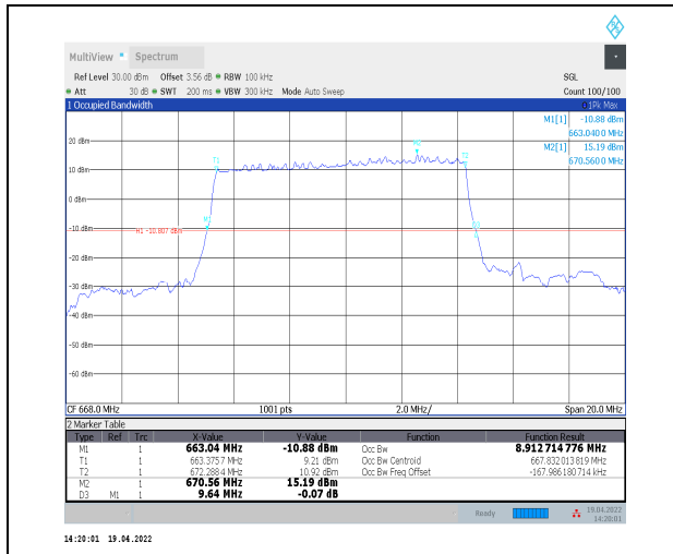
1-N71--15-10-L-2-DFT-PI2BPSK-Outer_Full-50@0-A nt0-8.913-9.640-≤10-PASS
