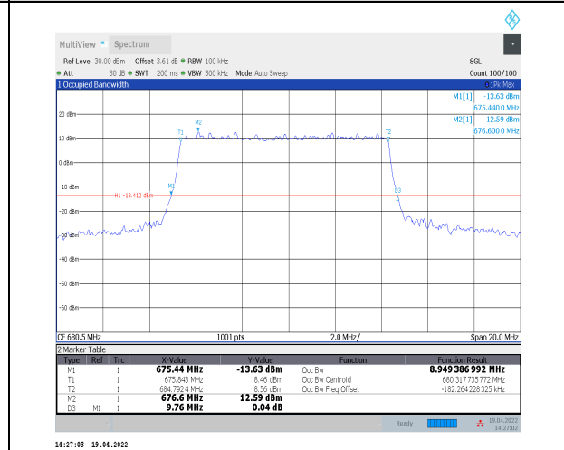
1-N71--15-10-M-4-DFT-64QAM-Outer_Full-50@0-A nt0-8.949-9.760≤10-PASS
