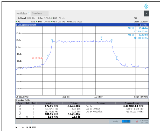
1-N71--15-5-M-8-CP-64QAM-Outer_Full-25@0-Ant0 -4.493-5.190≤5-PASS
