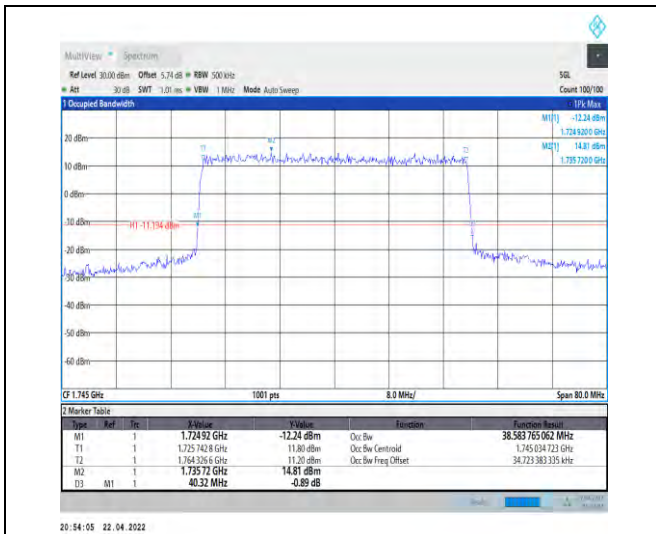
1-N66-PC3-15-40-M-1-DFT-QPSK-Outer_Full-216@ 0-Ant0-38.584-40.320-≤40-PASS
