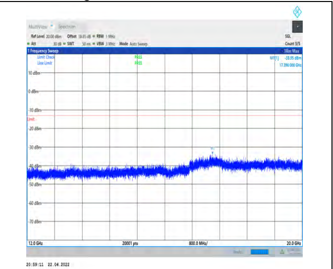
1-N66-PC3-15-40-L-1-DFT-PI2BPSK-Inner_1RB_Lef t-1@1-12000-20000-Ant0--33.95--13-PASS
