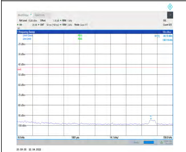
1-N66-PC3-15-40-M-1-DFT-PI2BPSK-Inner_1RB_L eft-1@1-0.009-0.15-Ant0--94.19--43-PASS
