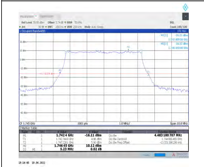
1-N66-PC3-15-5-M-6-CP-QPSK-Outer_Full-25@0-Ant0-4.483-5.230-≤5-PASS
