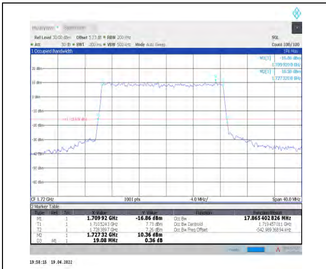
1-N66-PC3-15-20-L-4-DFT-64QAM-Outer_Full-100 @0-Ant0-17.865-19.080-≤20-PASS
