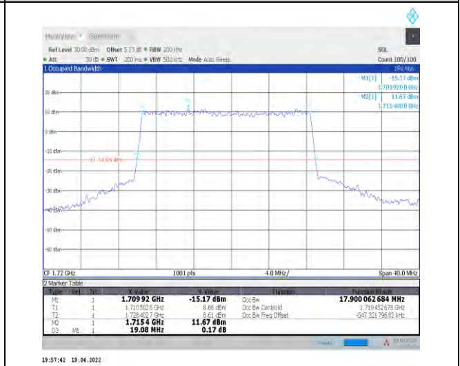
1-N66-PC3-15-20-L-3-DFT-16QAM-Outer_Full-100 @0-Ant0-17.9-19.080-≤20-PASS
