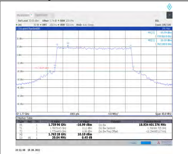
1-N66-PC3-15-20-H-7-CP-16QAM-Outer_Full-106@0 0-Ant0-18.934-20.040-≤20-PASS
