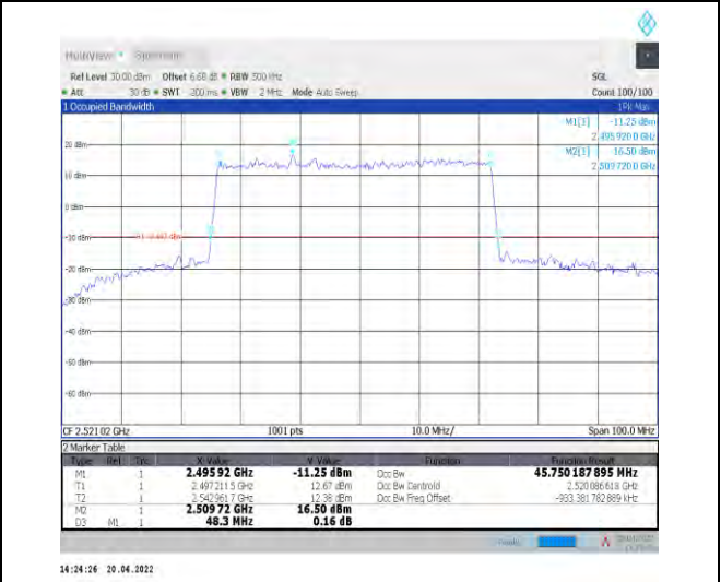
1-N41--30-50-L-3-DFT-16QAM-Outer_Full-128@0-A nt0-45.75-48.300-≤50-PASS
