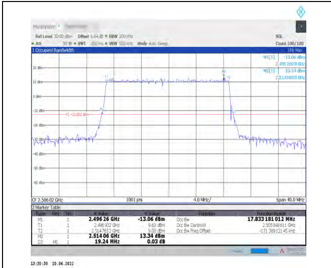
1-N41--30-20-L-5-DFT-256QAM-Outer_Full-50@0-A nt0-17.833-19.240-≤20-PASS
