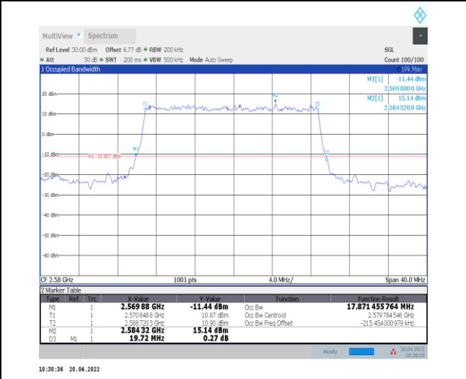
1-N38--30-20-L-2-DFT-PI2BPSK-Outer_Full-50@0-Ant0 nt0-17.871-19.720≤20-PASS
