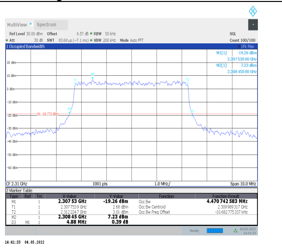
1-N30--15-5-M-9-CP-256QAM-Outer_Full-25@0-Ant 0-4.471-4.880-≤5-PASS
