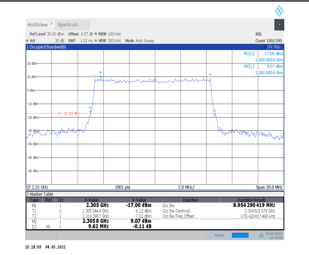
1-N30--15-10-L-5-DFT-256QAM-Outer_Full-50@0-A nt0-8.954-9.620≤10-PASS
