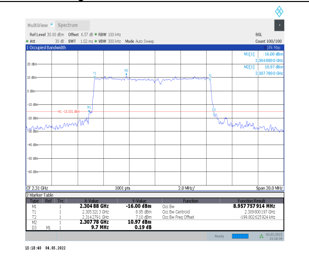
1-N30--15-10-L-3-DFT-16QAM-Outer_Full-50@0-Ant 0-8.958-9.700≤10-PASS
