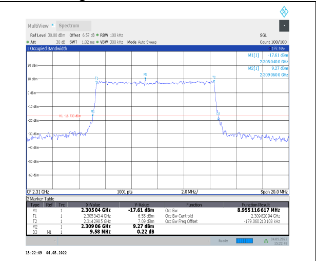
1-N30--15-10-H-5-DFT-256QAM-Outer_Full-50@0-A nt0-8.955-9.580-≤10-PASS
