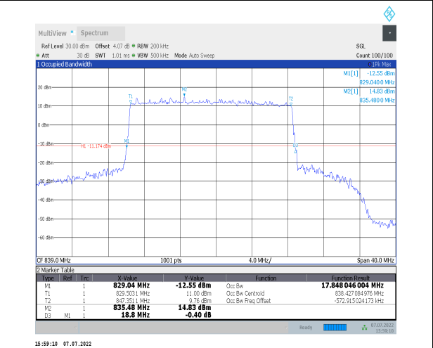
1-N26-824-849--15-20-H-1-DFT-QPSK-Outer_Full-1 00@0-Ant0-17.848-18.800-≤20-PASS
