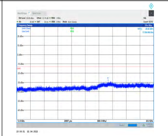
1-N25--15-40-M-1-DFT-PI2BPSK-Inner_1RB_Left-1 @1-12000-20000-Ant0--28.62--13-PASS
