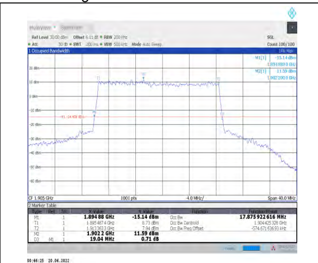
1-N25--15-20-H-3-DFT-16QAM-Outer_Full-100@0-Ant0-17.876-19.040-≤20-PASS
