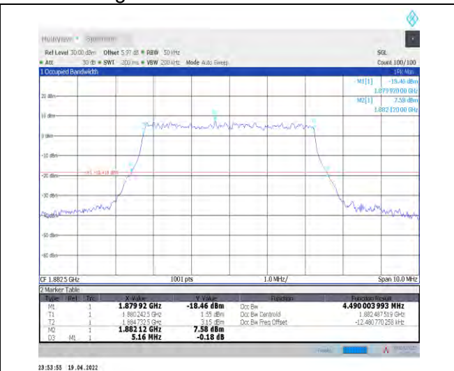
1-N25--15-5-M-9-CP-256QAM-Outer_Full-25@0-Ant0 0-4.49-5.160-≤5-PASS
