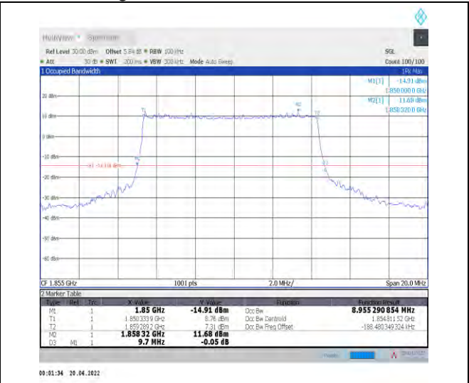
1-N25--15-10-L-3-DFT-16QAM-Outer_Full-50@0-Ant 0-8.955-9.700-≤10-PASS
