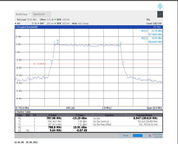
1-N14--15-10-L-5-DFT-256QAM-Outer_Full-50@0-A nt0-8.947-9.640≤10-PASS
