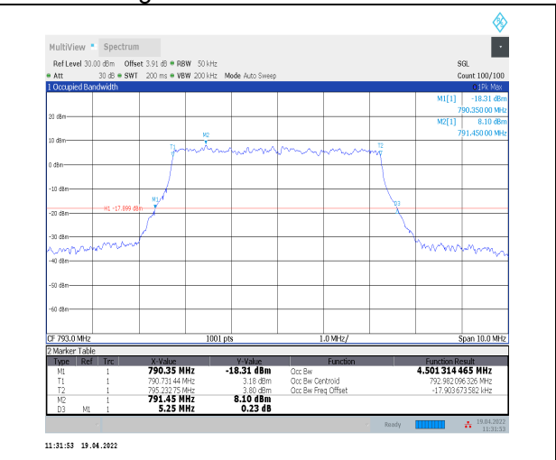
1-N14--15-5-M-9-CP-256QAM-Outer_Full-25@0-Ant 0-4.501-5.250-≤5-PASS
