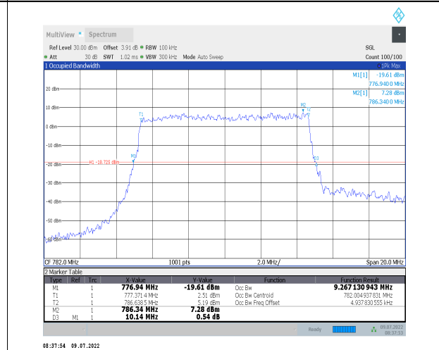
1-N13--15-10-M-9-CP-256QAM-Outer_Full-52@0-Ant0-9.267-10.140-≤10-PASS
