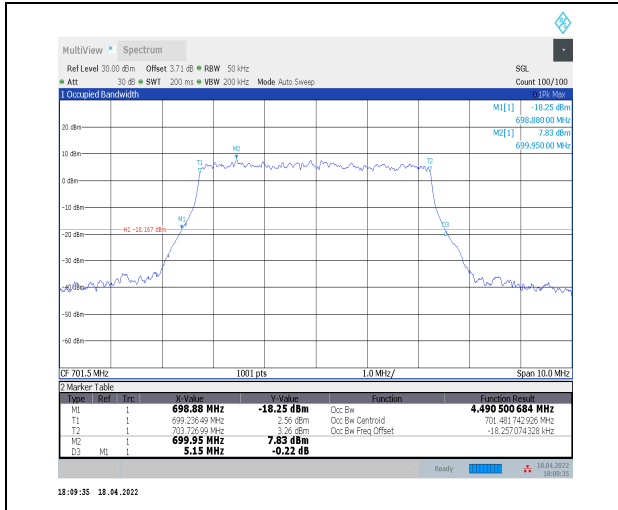
1-N12--15-5-L-9-CP-256QAM-Outer_Full-25@0-Ant0 -4.491-5.150-≤5-PASS
