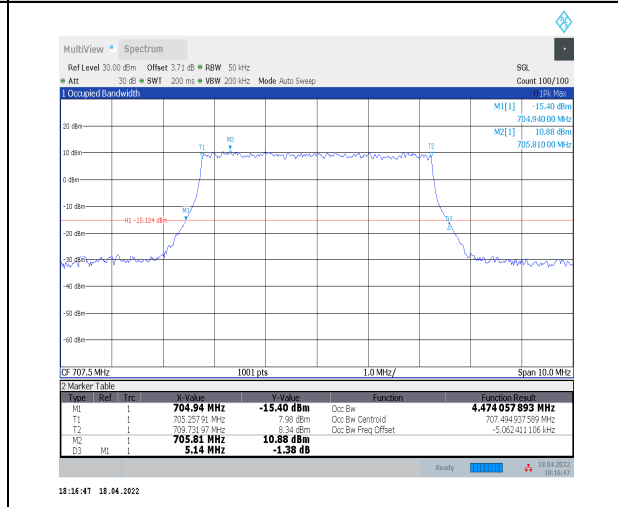
1-N12--15-5-M-7-CP-16QAM-Outer_Full-25@0-Ant0 -4.474-5.140-≤5-PASS
