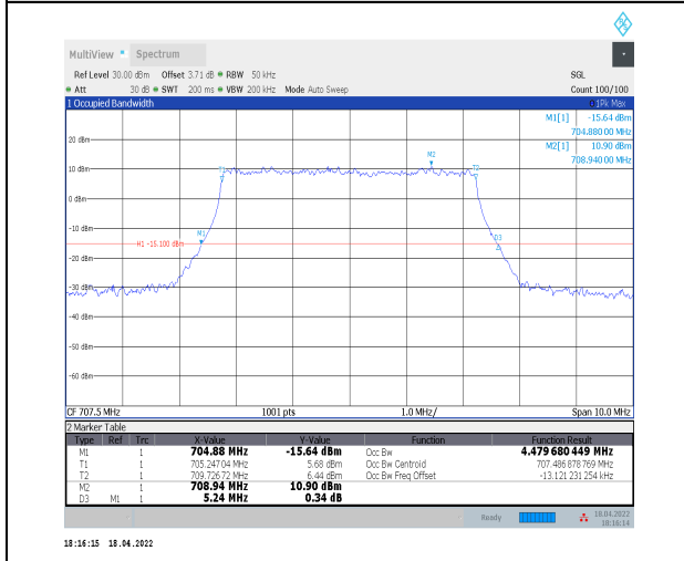
1-N12--15-5-M-6-CP-QPSK-Outer_Full-25@0-Ant0-4 .48-5.240-≤5-PASS
