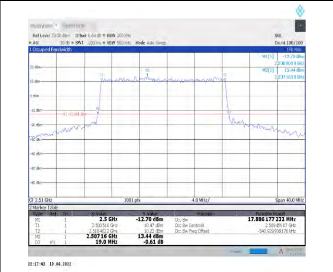
1-N7--15-20-L-3-DFT-16QAM-Outer_Full-100@0-Ant 0-17.886-19.000-≤20-PASS
