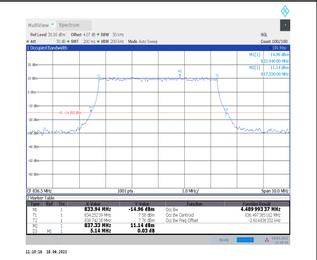
1-N5--15-5-M-7-CP-16QAM-Outer_Full-25@0-Ant0- 4.49-5.140≤5-PASS
