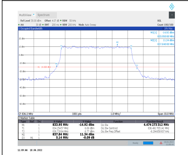
1-N5--15-5-M-6-CP-QPSK-Outer_Full-25@0-Ant0-4. 474-5.140≤5-PASS
