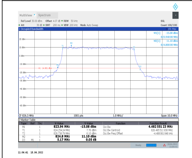
1-N5--15-5-L-7-CP-16QAM-Outer_Full-25@0-Ant0-4 .483-5.170-≤5-PASS
