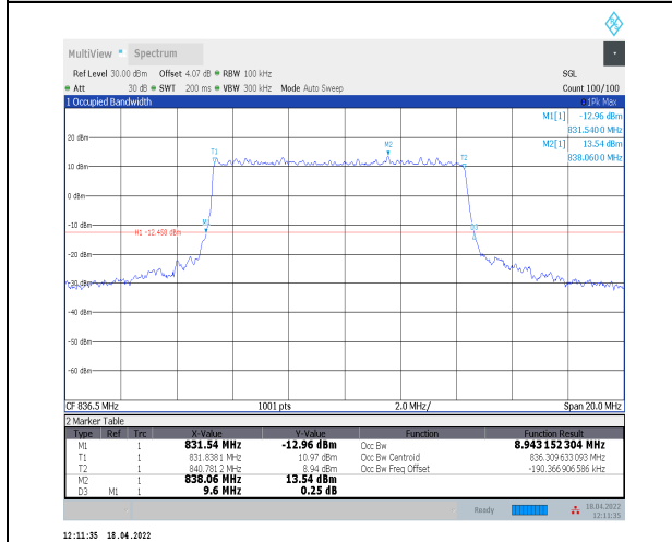
1-N5--15-10-M-3-DFT-16QAM-Outer_Full-50@0-Ant0 0-8.943-9.600-≤10-PASS
