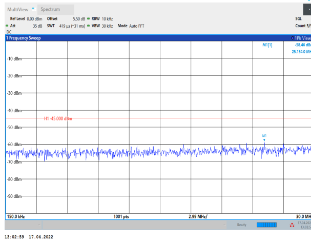
Band41-20MHz-QPSK-39750-1RB#0-Range2:0.15~30MHz
