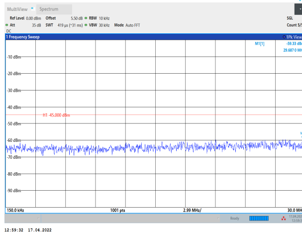
Band38-20MHz-QPSK-37850-1RB#0-Range2:0.15~30MHz
