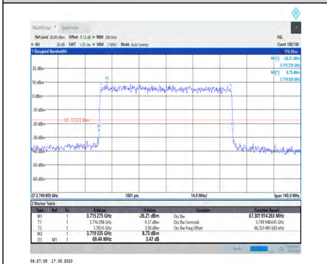
1-N78-3700-3800-PC1-30-70-M-9-CP-256QAM-Outer _Full-189@0-Ant1-67.302-69.440-≤70-PASS
