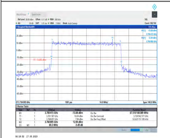
1-N78-3700-3800-PC1-30-70-L-6-CP-QPSK-Outer_Full-189@0-Ant1-67.51-69.300-≤70-PASS
