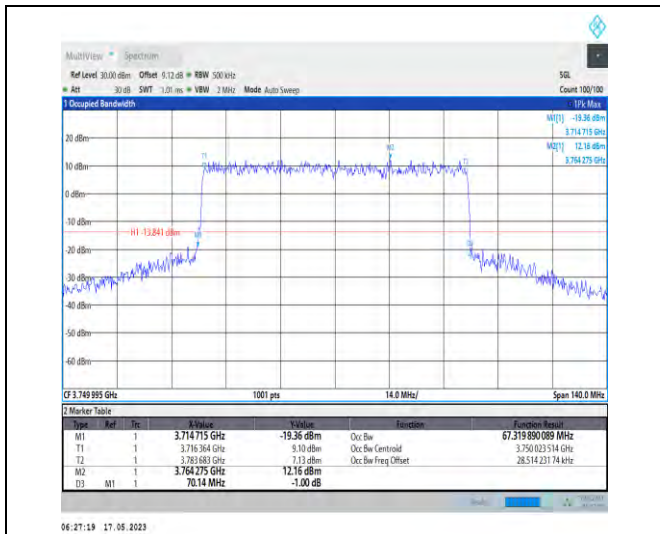
1-N78-3700-3800-PC1-30-70-M-7-CP-16QAM-Outer _Full-189@0-Ant1-67.32-70.140-≤70-PASS
