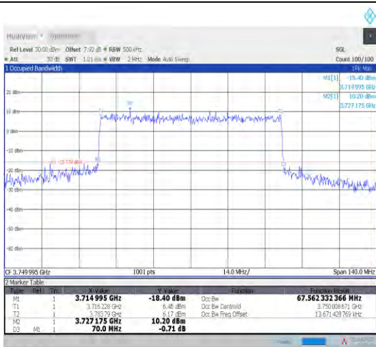
1-N78-3700-3800--30-70-M-7-CP-16QAM-Outer_Full -189@0-Ant1-67.562-70.000-≤70-PASS
