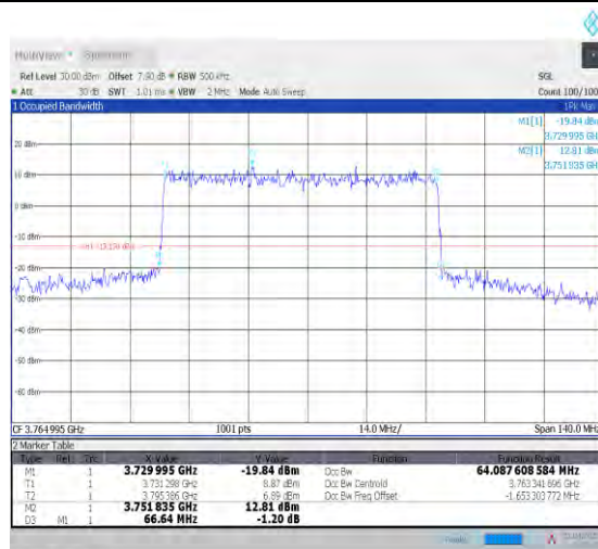
1-N78-3700-3800--30-70-M-8-CP-64QAM-Outer_Ful I-189@0-Ant1-67.508-69.860-≤70-PASS
