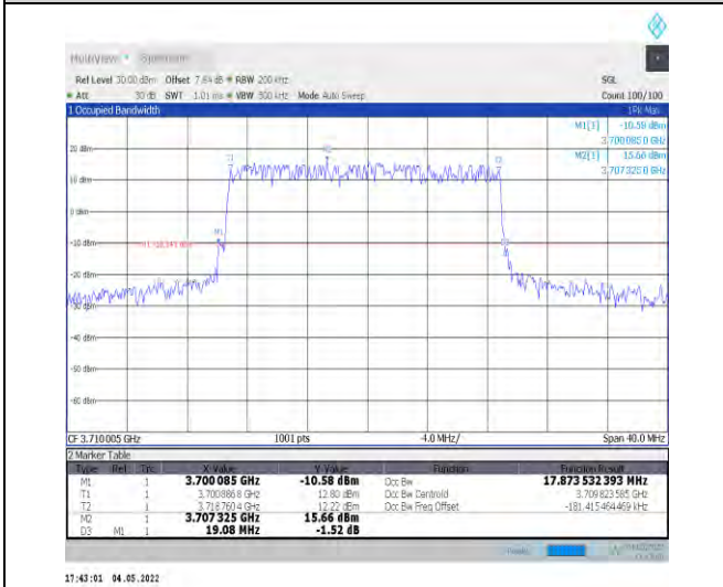
1-N78-3700-3800--30-20-L-1-DFT-QPSK-Outer_Full -50@0-Ant1-17.874-19.080-≤20-PASS
