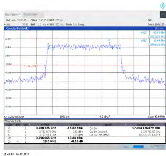
1-N78-3700-3800--30-20-H-4-DFT-64QAM-Outer_Fu II-50@0-Ant1-17.904-19.000-≤20-PASS
