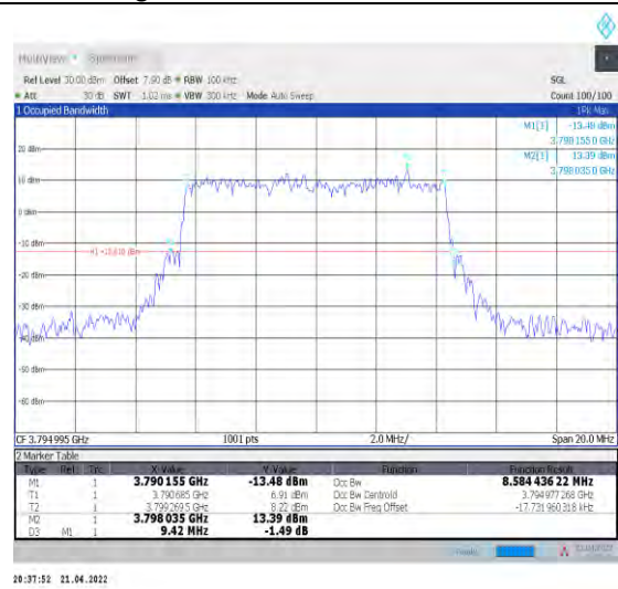
1-N78-3700-3800--30-10-H-4-DFT-64QAM-Outer_Fu II-24@0-Ant1-8.584-9.420-≤10-PASS
