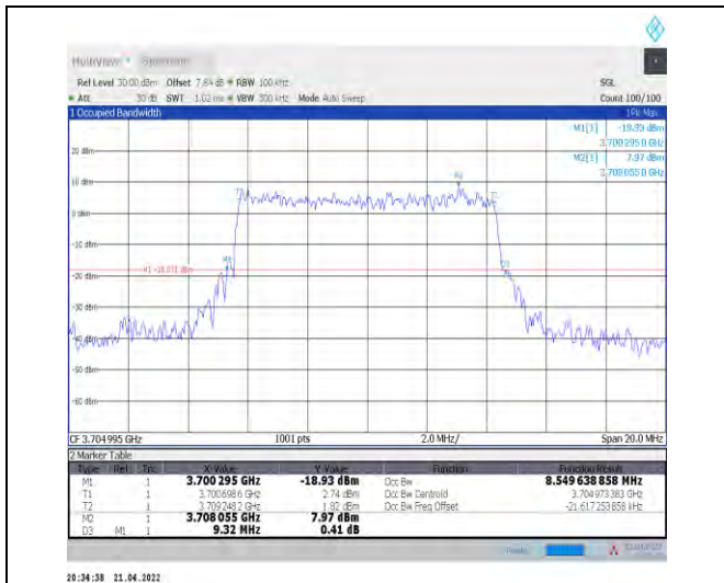
1-N78-3700-3800--30-10-L-9-CP-256QAM-Outer_Fu II-24@0-Ant1-8.55-9.320-≤10-PASS
