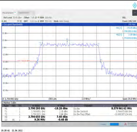
1-N78-3700-3800--30-10-H-9-CP-256QAM-Outer_Fu II-24@0-Ant1-8.58-9.360-≤10-PASS
