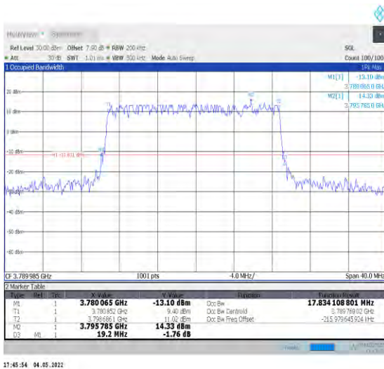
1-N78-3700-3800--30-20-H-3-DFT-16QAM-Outer_Fu II-50@0-Ant1-17.834-19.200-≤20-PASS
