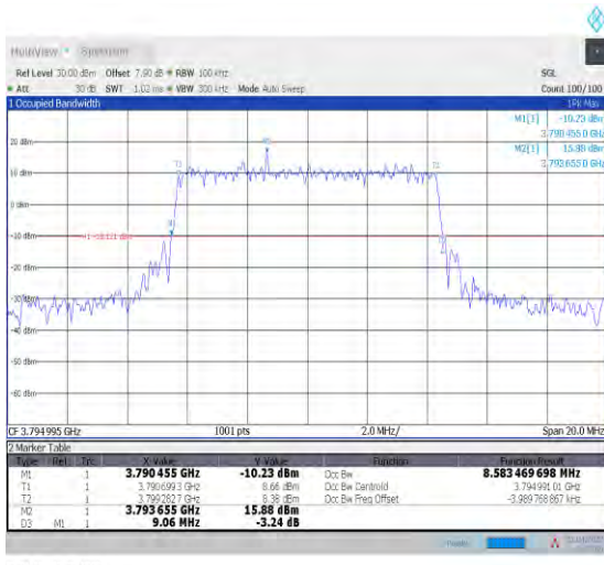
1-N78-3700-3800--30-10-H-1-DFT-QPSK-Outer_Full -24@0-Ant1-8.583-9.060-≤10-PASS
