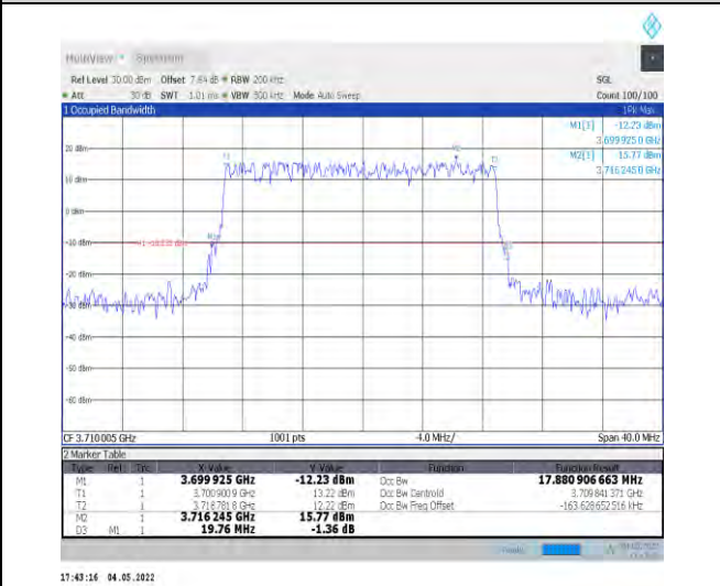
1-N78-3700-3800--30-20-L-2-DFT-PI2BPSK-Outer_Full -50@0-Ant1-17.881-19.760-≤20-PASS
