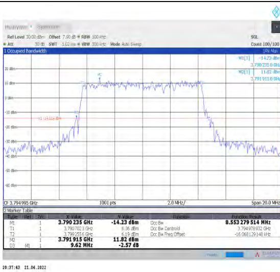
1-N78-3700-3800--30-10-H-3-DFT-16QAM-Outer_Fu II-24@0-Ant1-8.553-9.620-≤10-PASS
