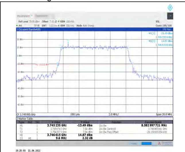
1-N78-3700-3800--30-10-M-1-DFT-QPSK-Outer_Full -24@0-Ant1-8.583-9.600-≤10-PASS
