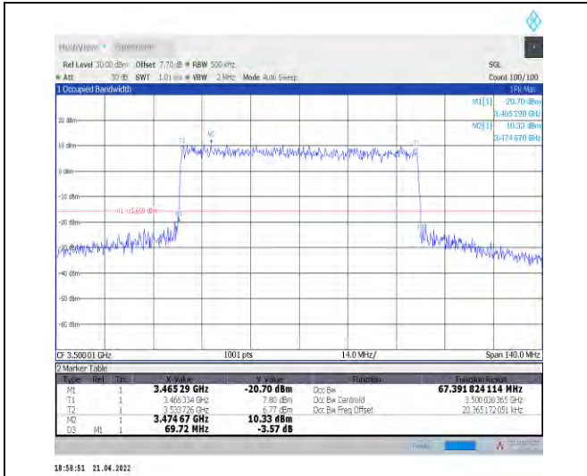
1-N78-3450-3550--30-70-M-7-CP-16QAM-Outer_Full -189@0-Ant1-67.392-69.720-≤70-PASS
