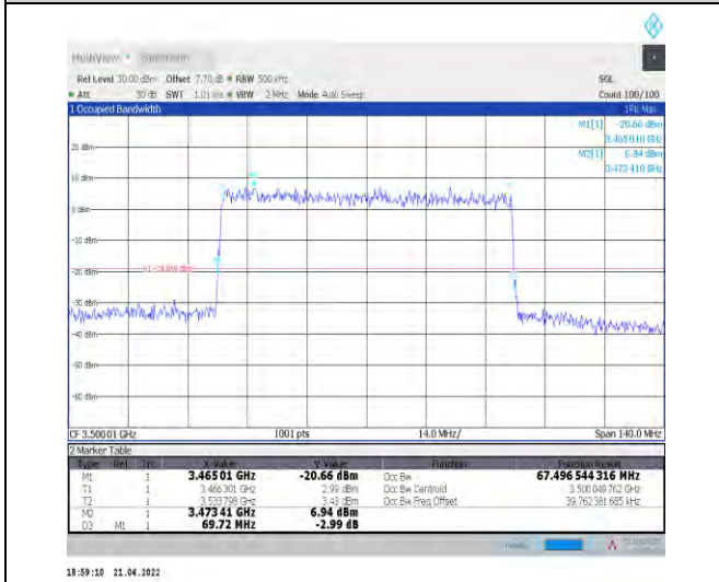
1-N78-3450-3550--30-70-M-9-CP-256QAM-Outer_F ull-189@0-Ant1-67.497-69.720-≤70-PASS
