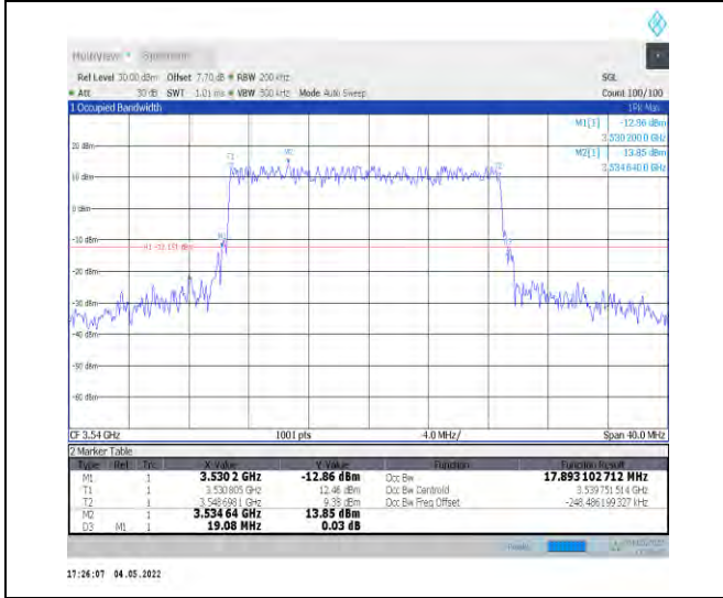
1-N78-3450-3550--30-20-H-3-DFT-16QAM-Outer_Fu II-50@0-Ant1-17.893-19.080-≤20-PASS
