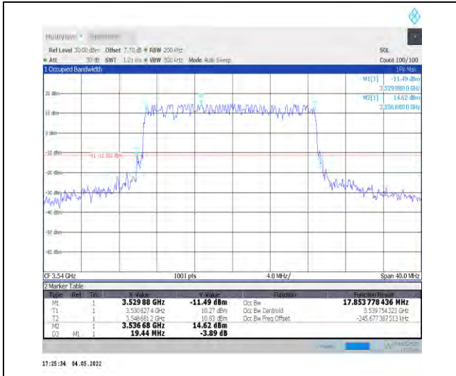
1-N78-3450-3550--30-20-H-1-DFT-QPSK-Outer_Full -50@0-Ant1-17.854-19.440-≤20-PASS
