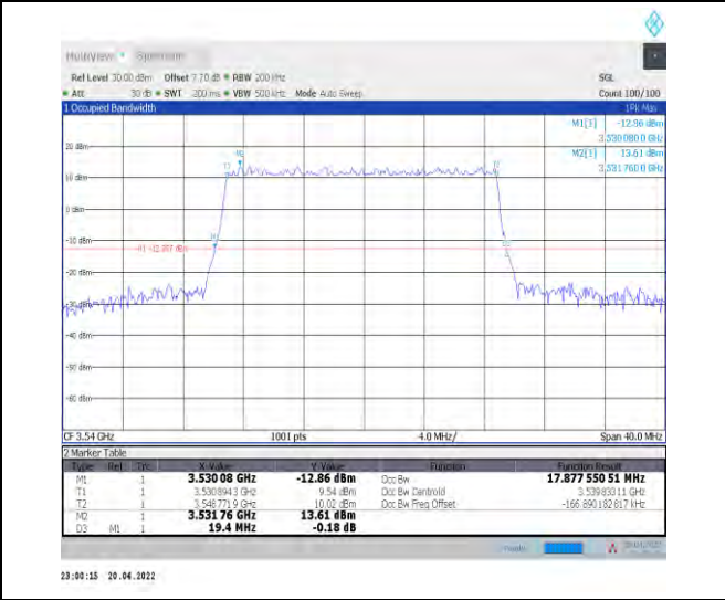
1-N78-3450-3550--30-20-H-4-DFT-64QAM-Outer_Fu II-50@0-Ant1-17.878-19.400-≤20-PASS
