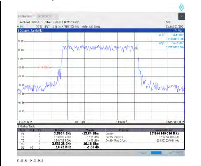
1-N78-3450-3550--30-20-H-2-DFT-PI2BPSK-Outer_Full -50@0-Ant1-17.844-18.720-≤20-PASS
