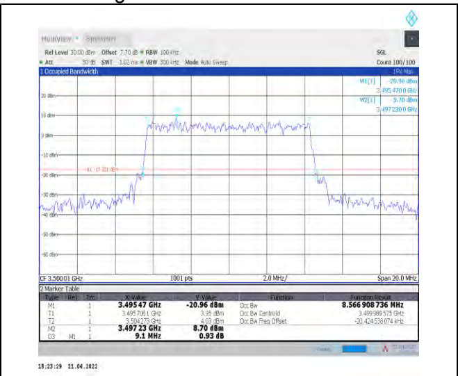
1-N78-3450-3550--30-10-M-9-CP-256QAM-Outer_Full -24@0-Ant1-8.567-9.100-≤10-PASS
