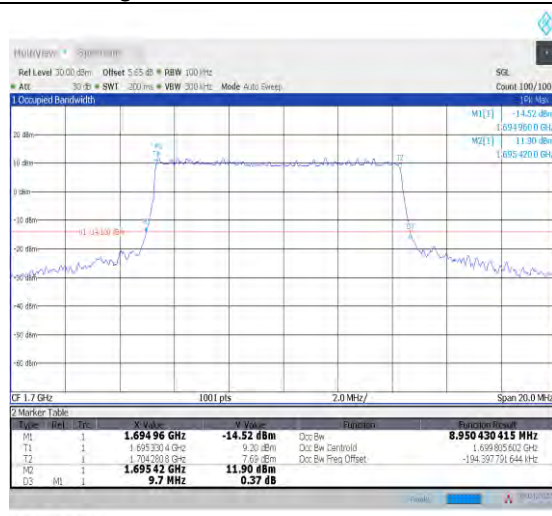
1-N70--15-10-L-3-DFT-16QAM-Outer_Full-50@0-An t1-8.95-9.700-≤10-PASS
